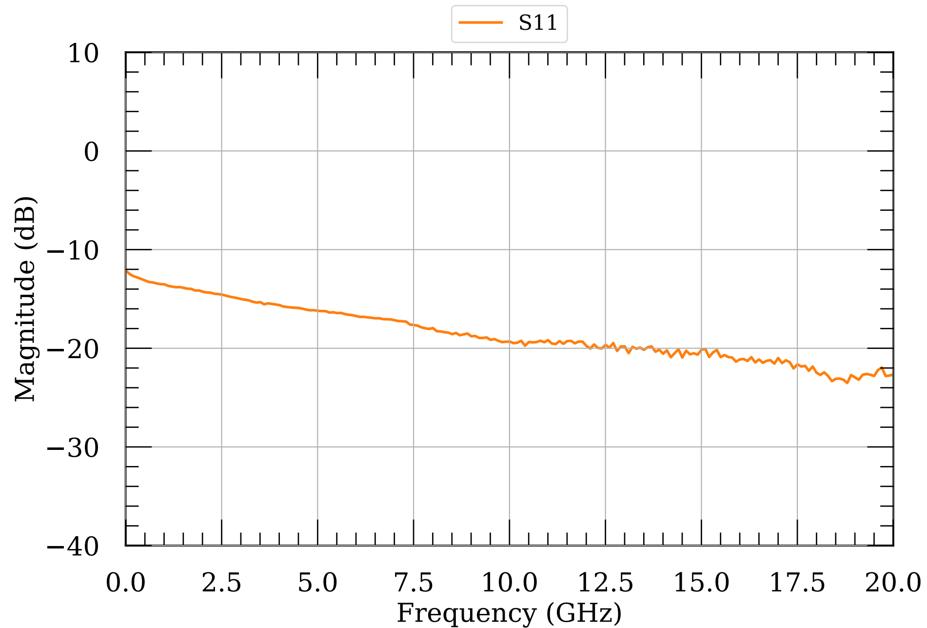
LNA S-params 10.5
