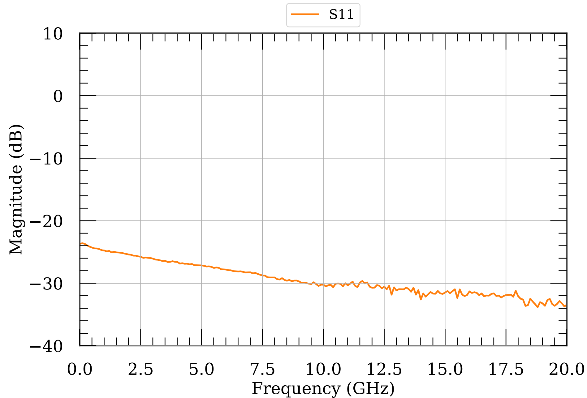
LNA S-params 21.0
