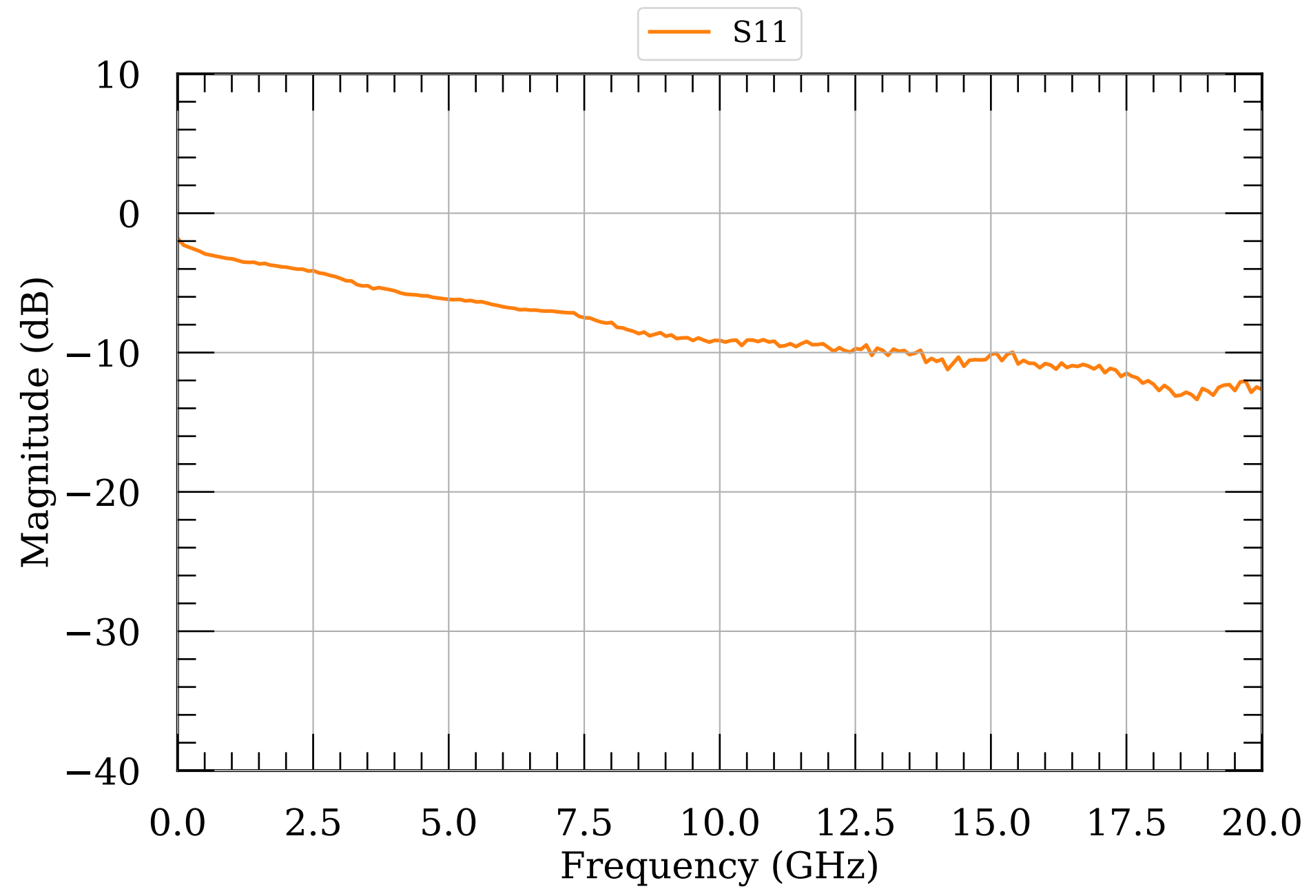
LNA S-params 05
