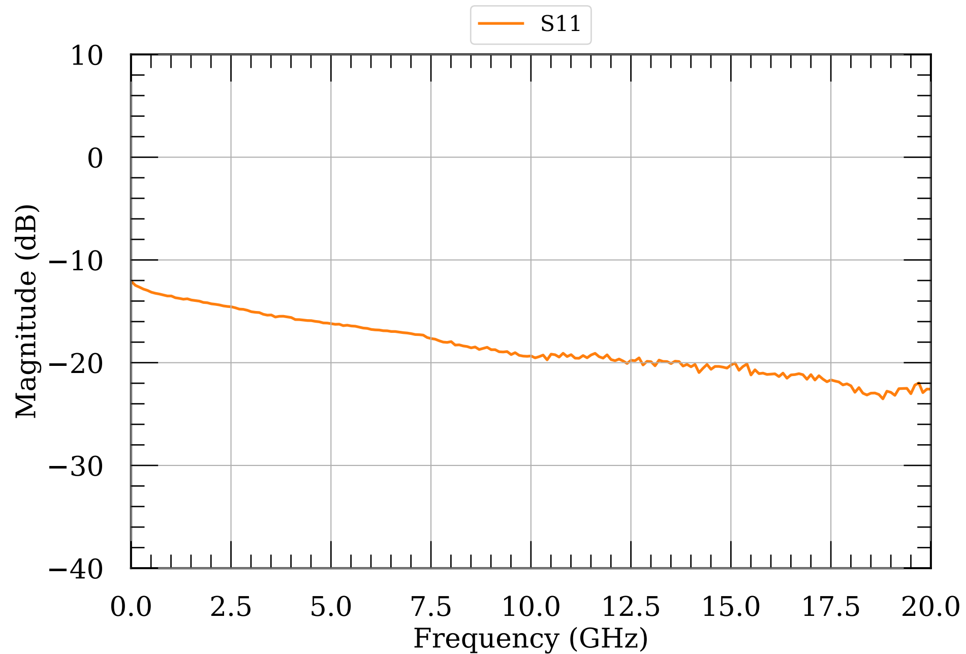
LNA S-params 100
