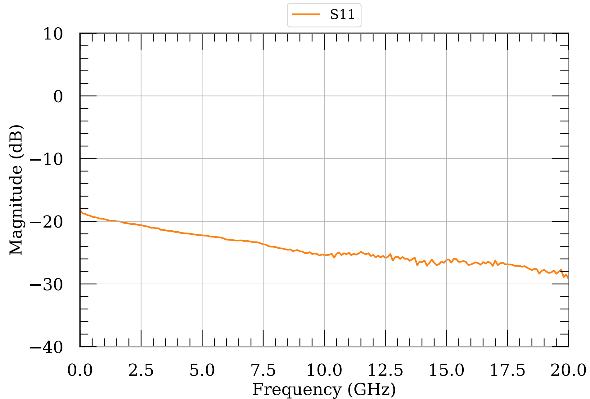
LNA S-params 10
