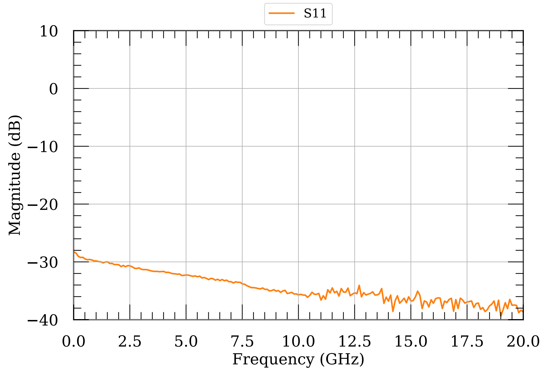
LNA S-params 110
