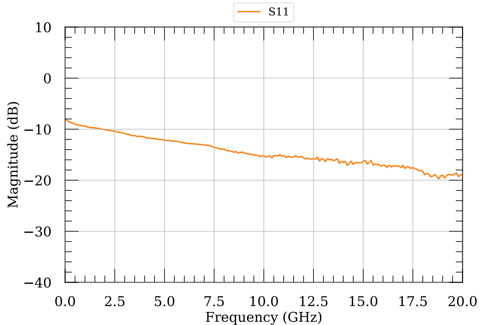
LNA S-params 120
