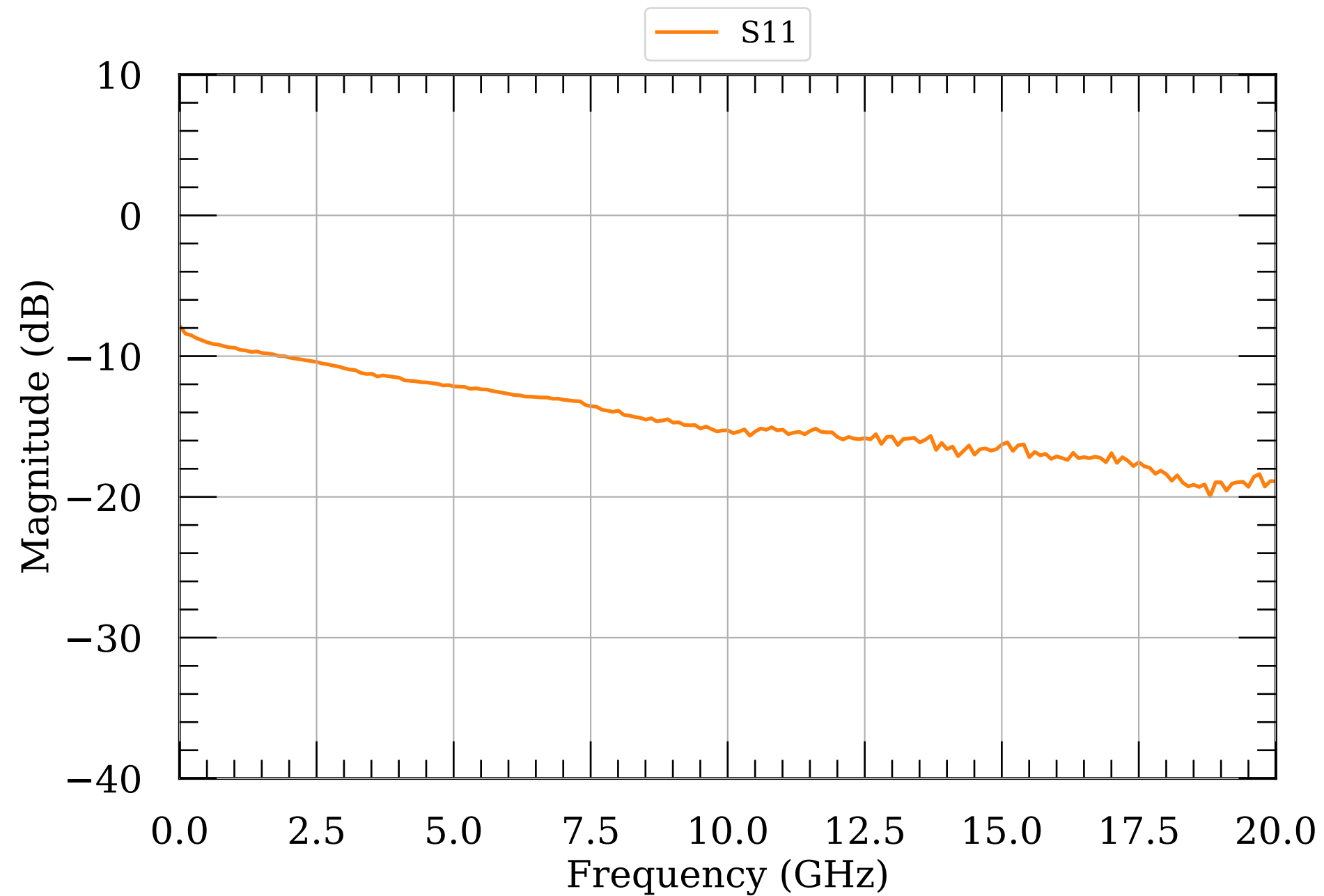
LNA S-params 125
