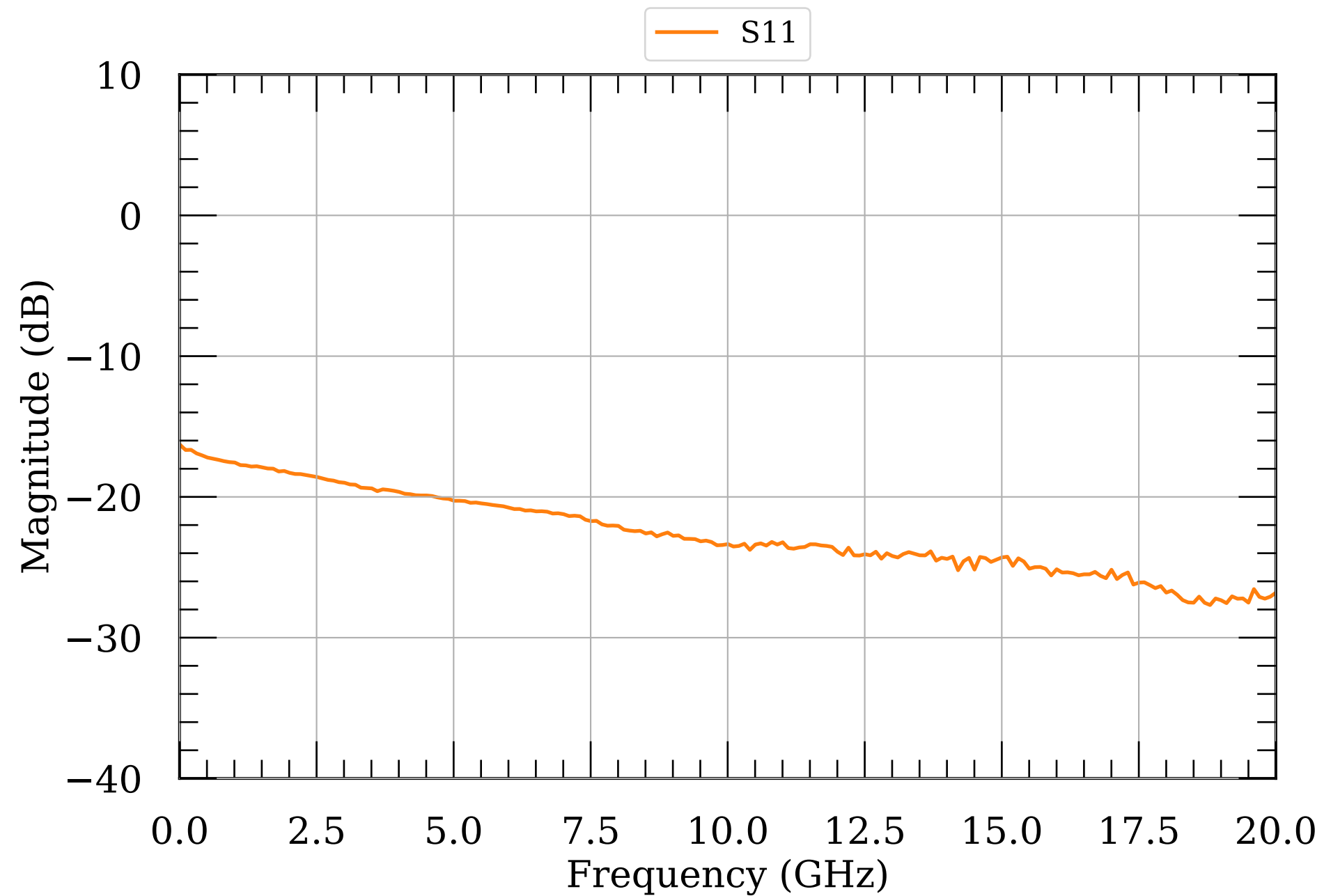
LNA S-params 140
