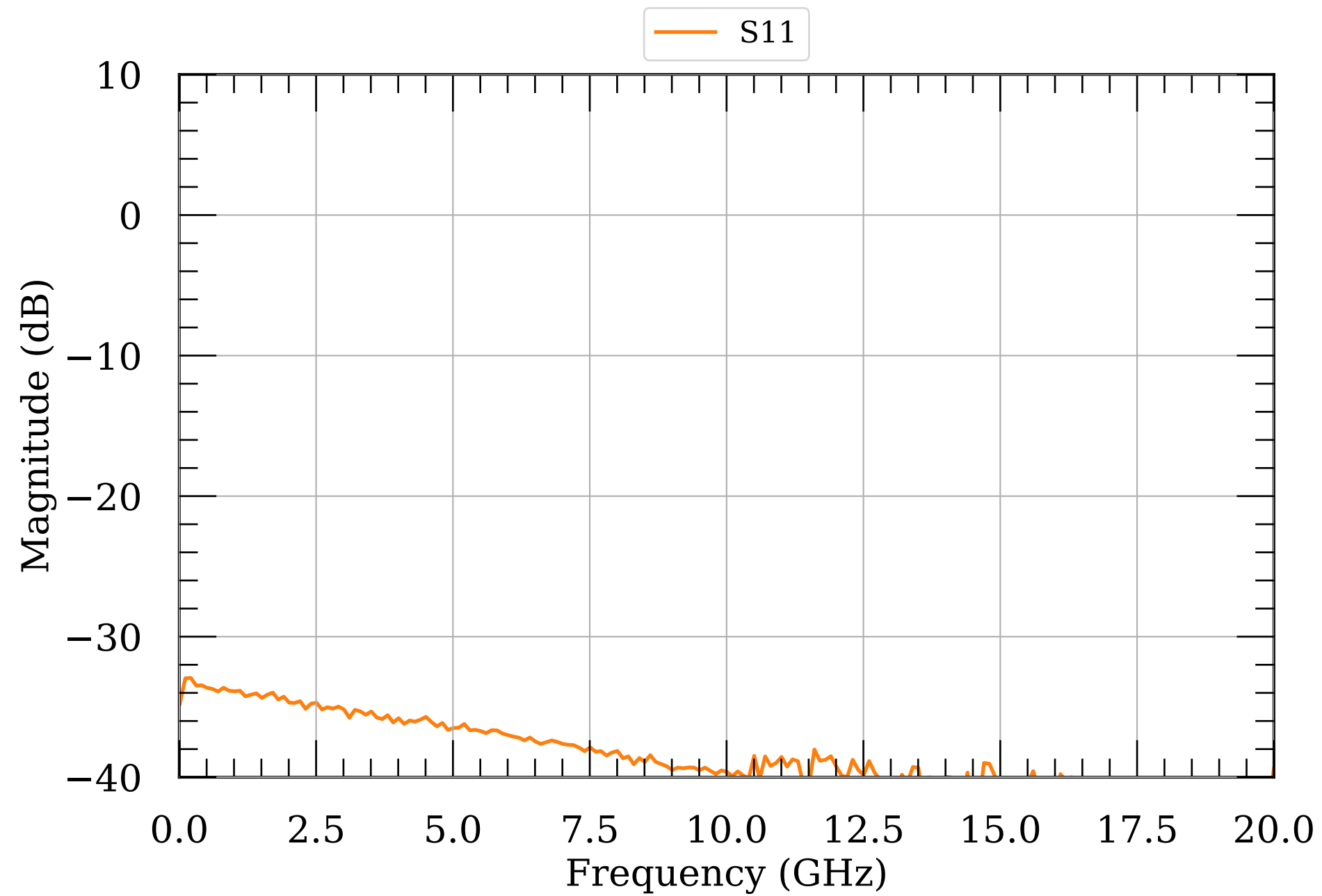
LNA S-params 150
