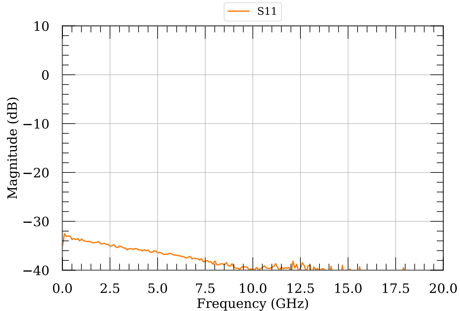
LNA S-params 155
