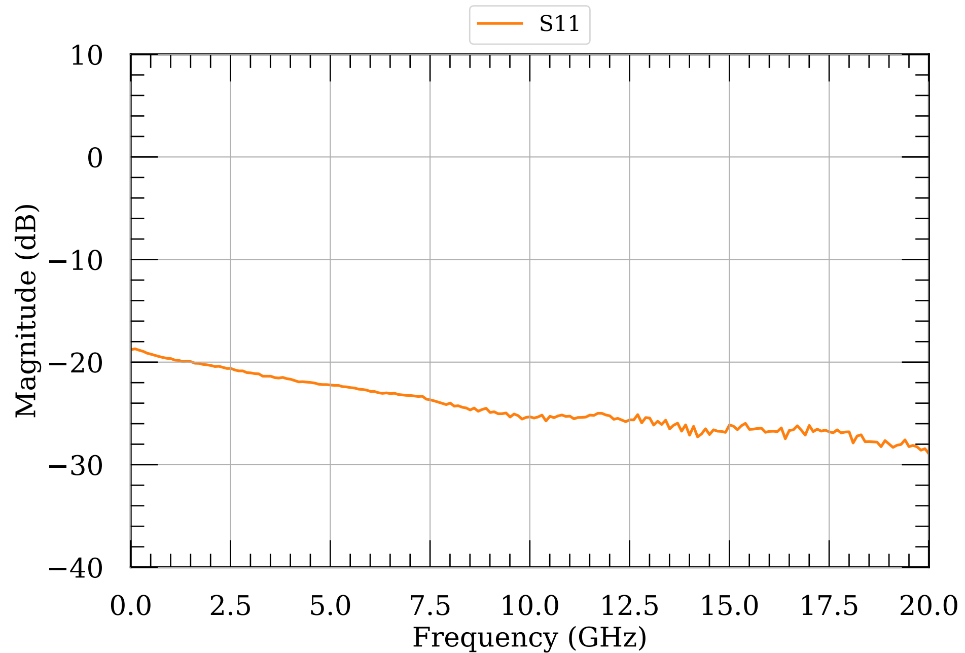
LNA S-params 15
