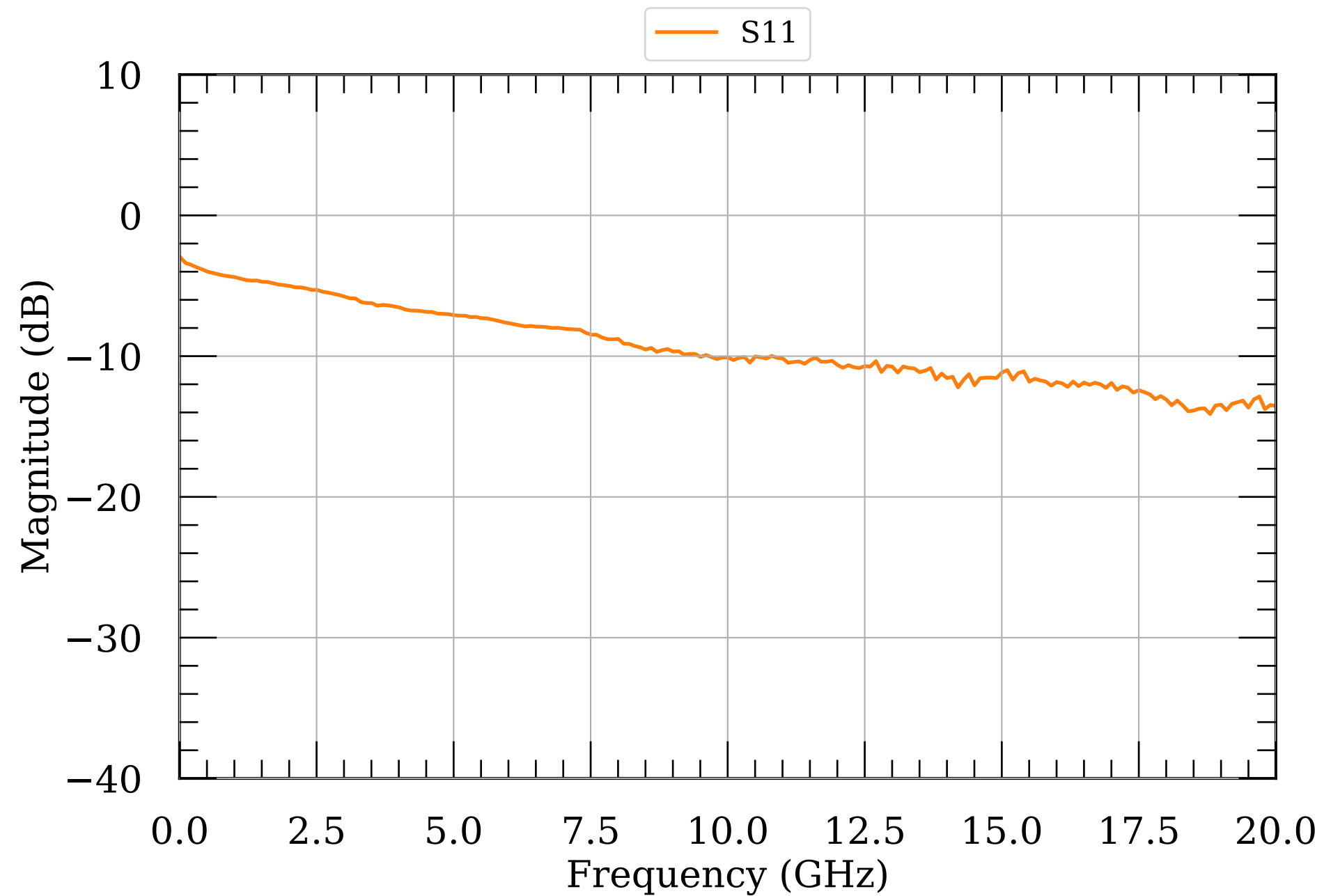
LNA S-params 160
