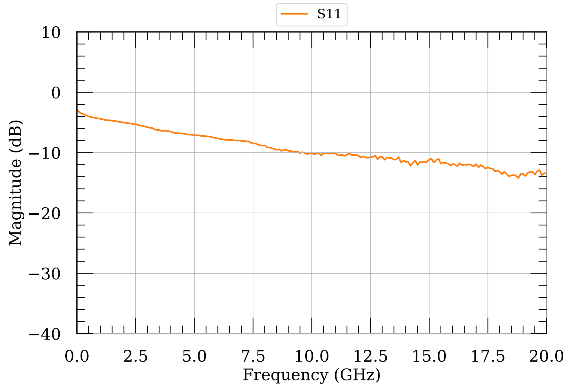
LNA S-params 165
