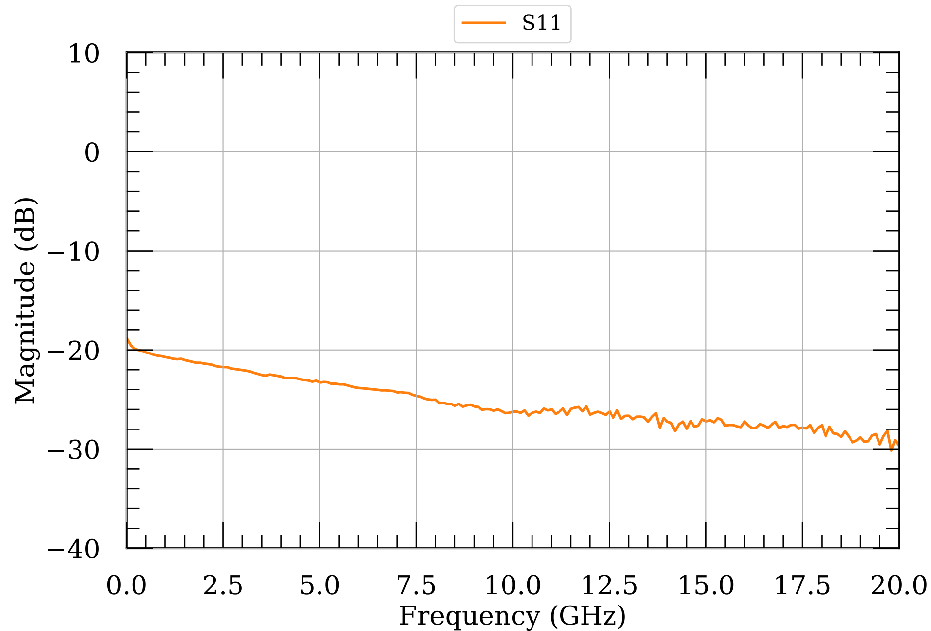
LNA S-params 175
