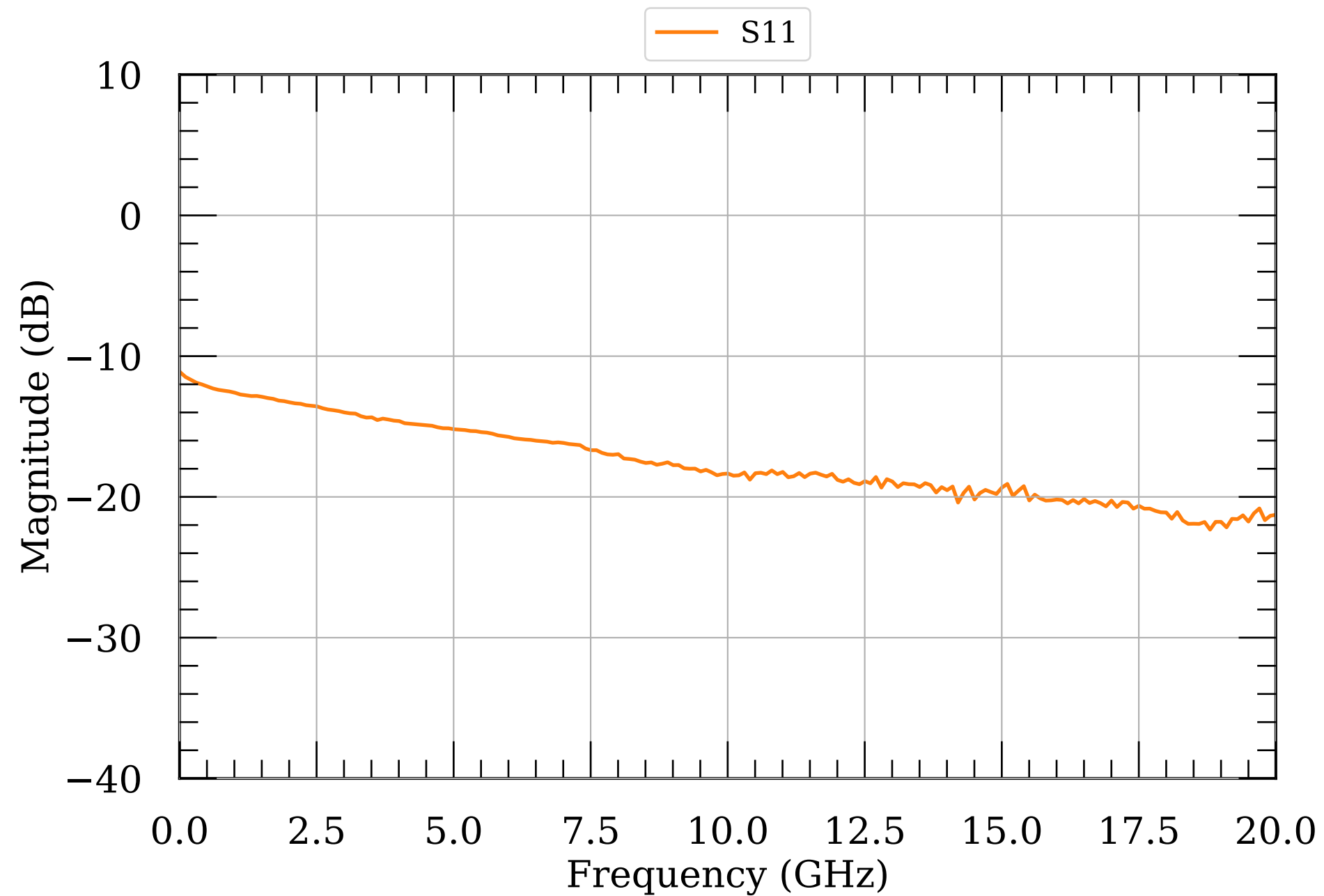
LNA S-params 180
