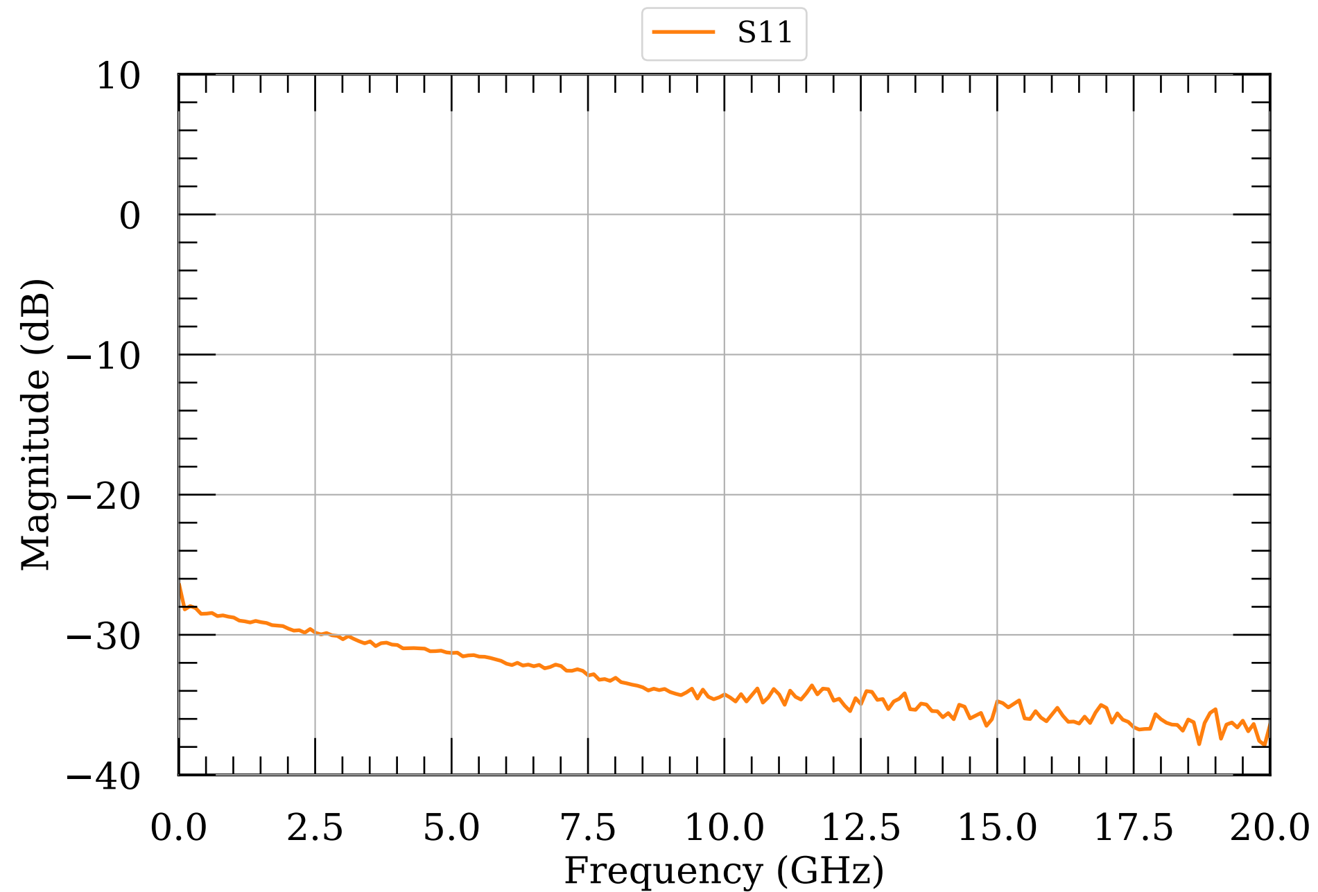
LNA S-params 190
