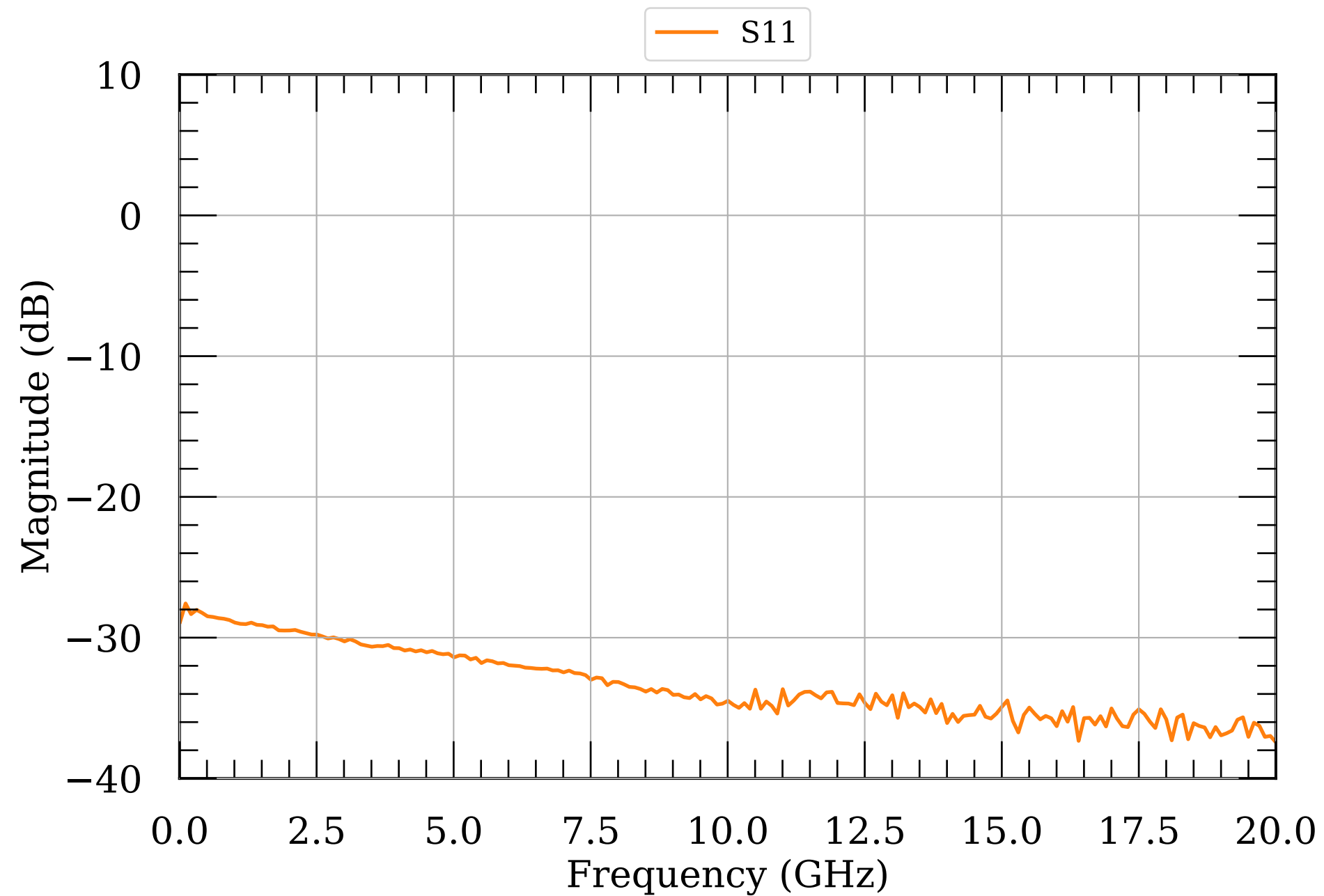
LNA S-params 195
