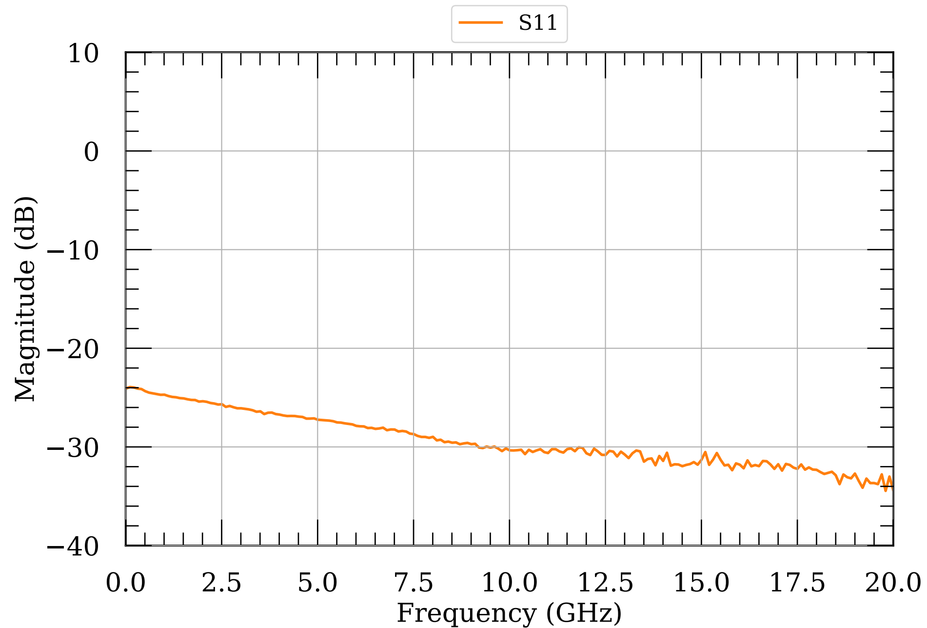
LNA S-params 215
