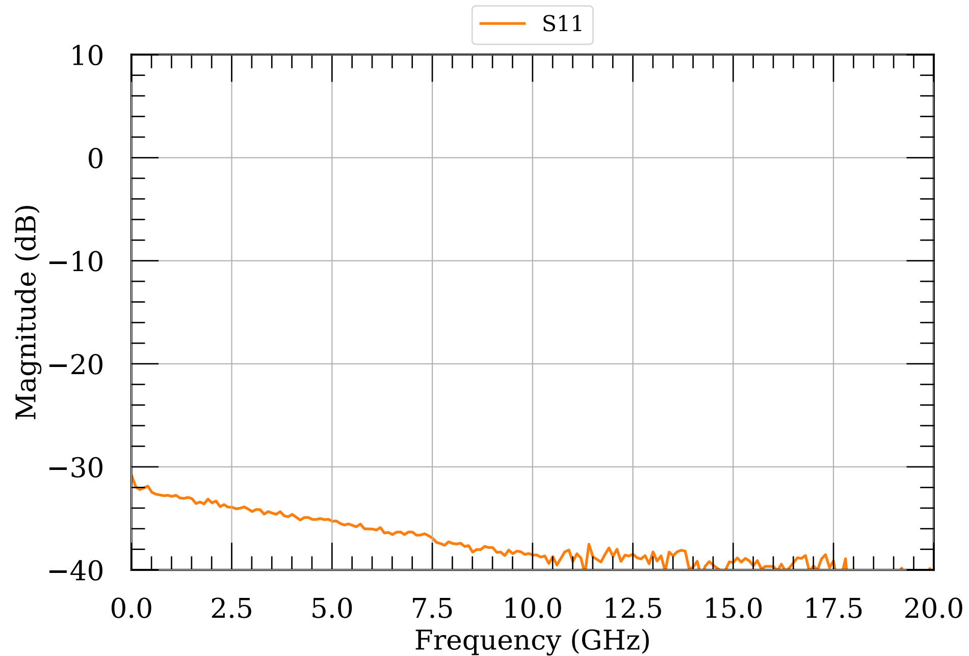
LNA S-params 230
