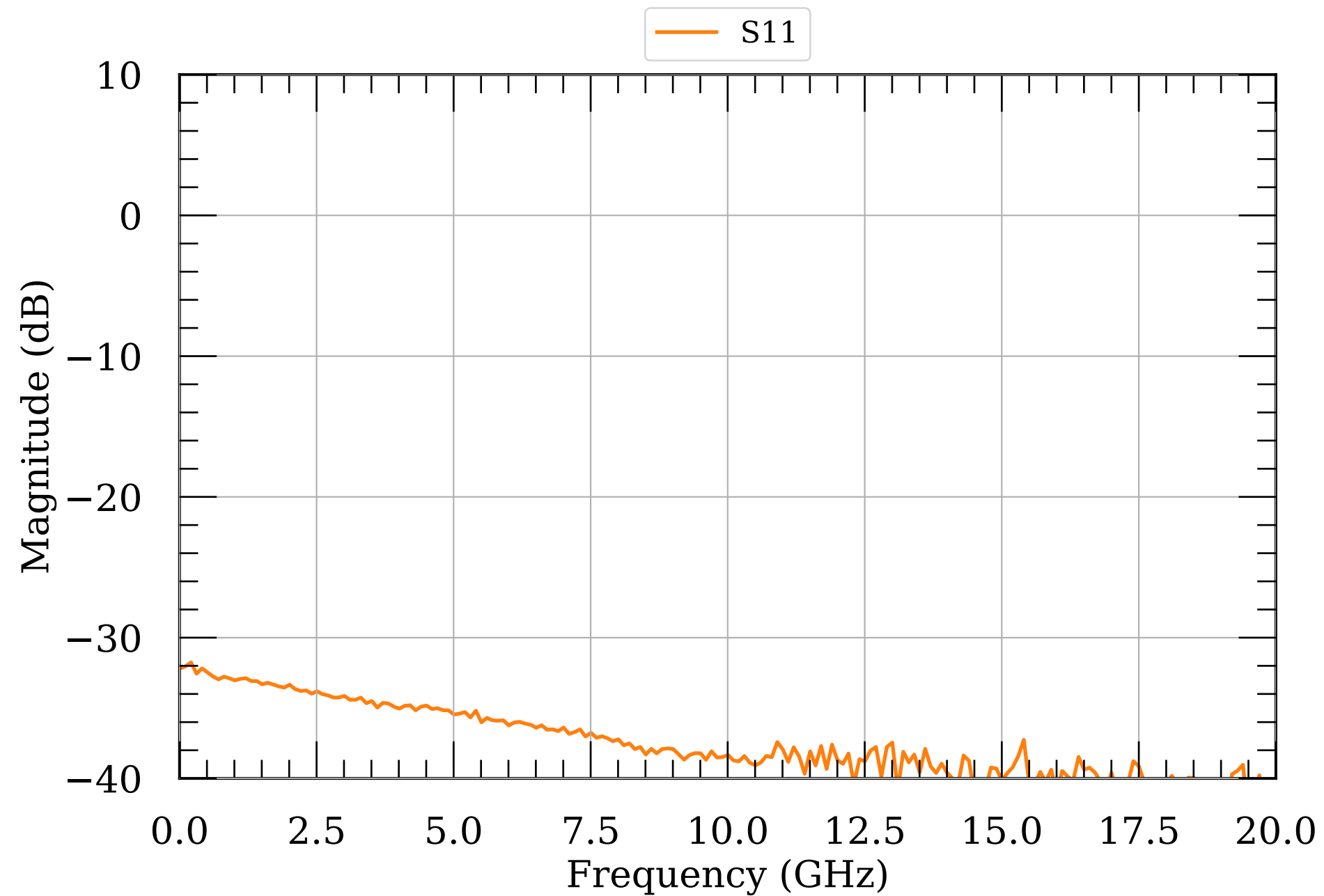
LNA S-params 235
