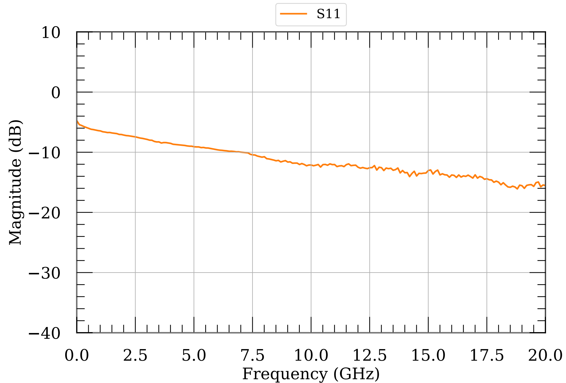
LNA S-params 245
