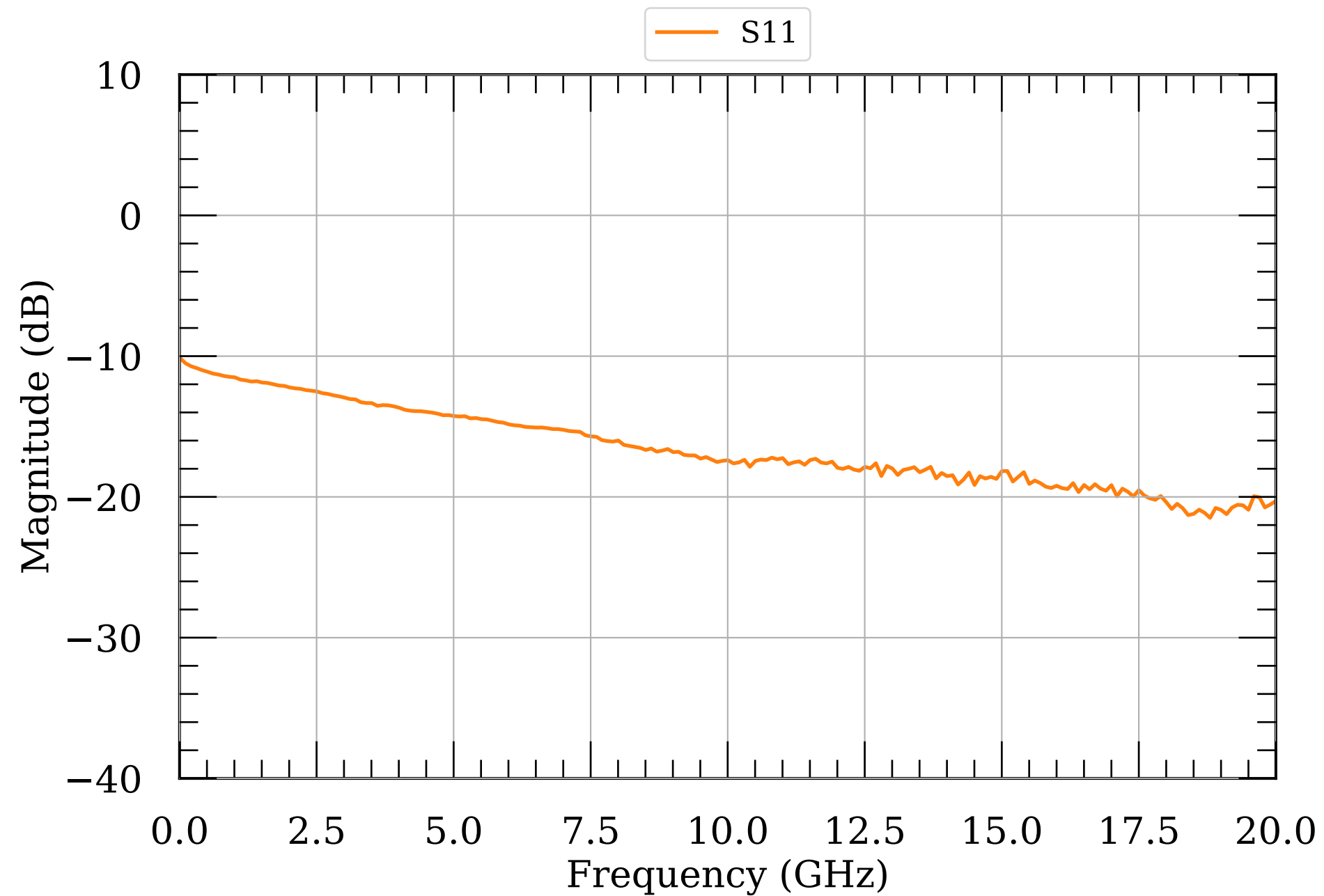
LNA S-params 25
