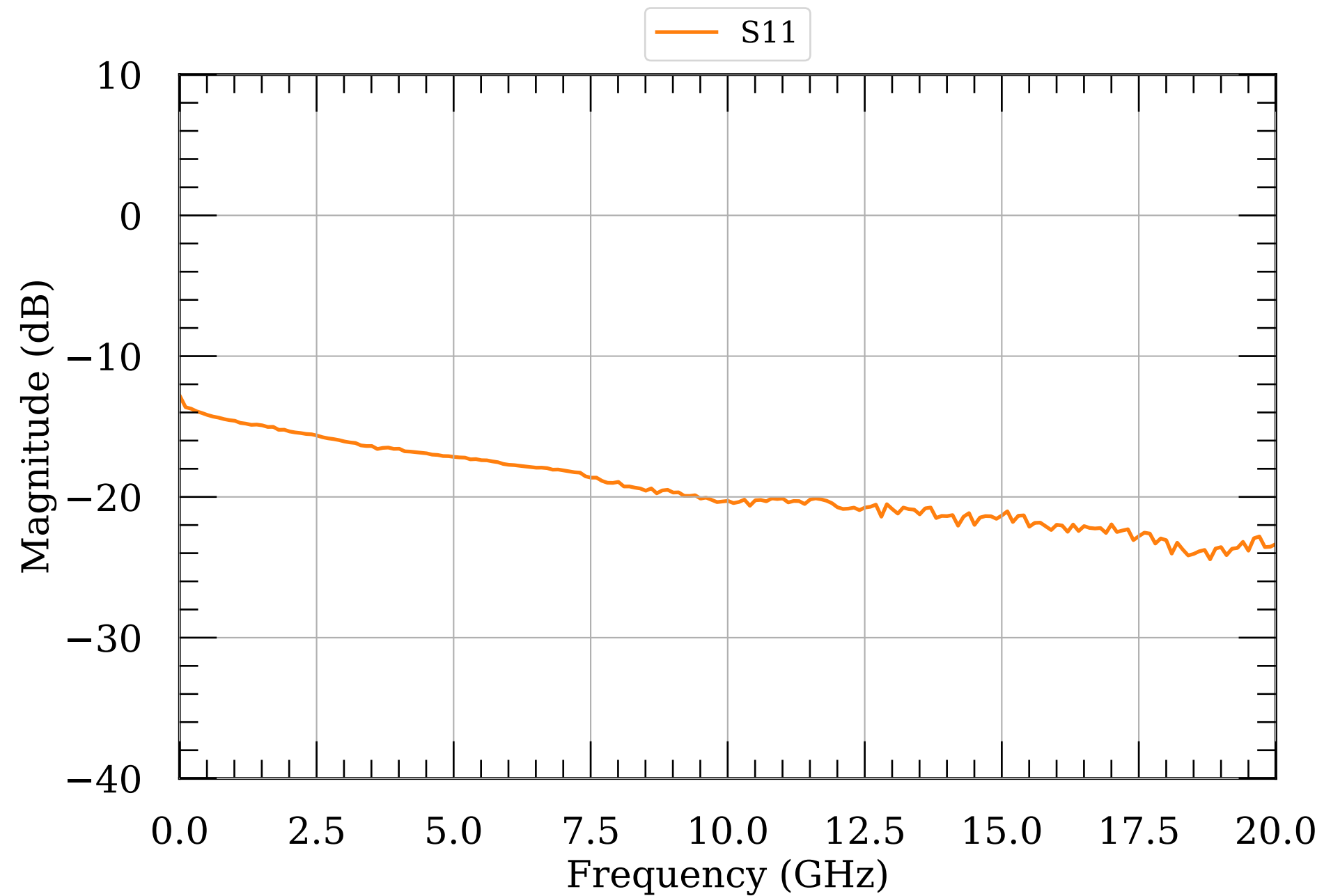
LNA S-params 260
