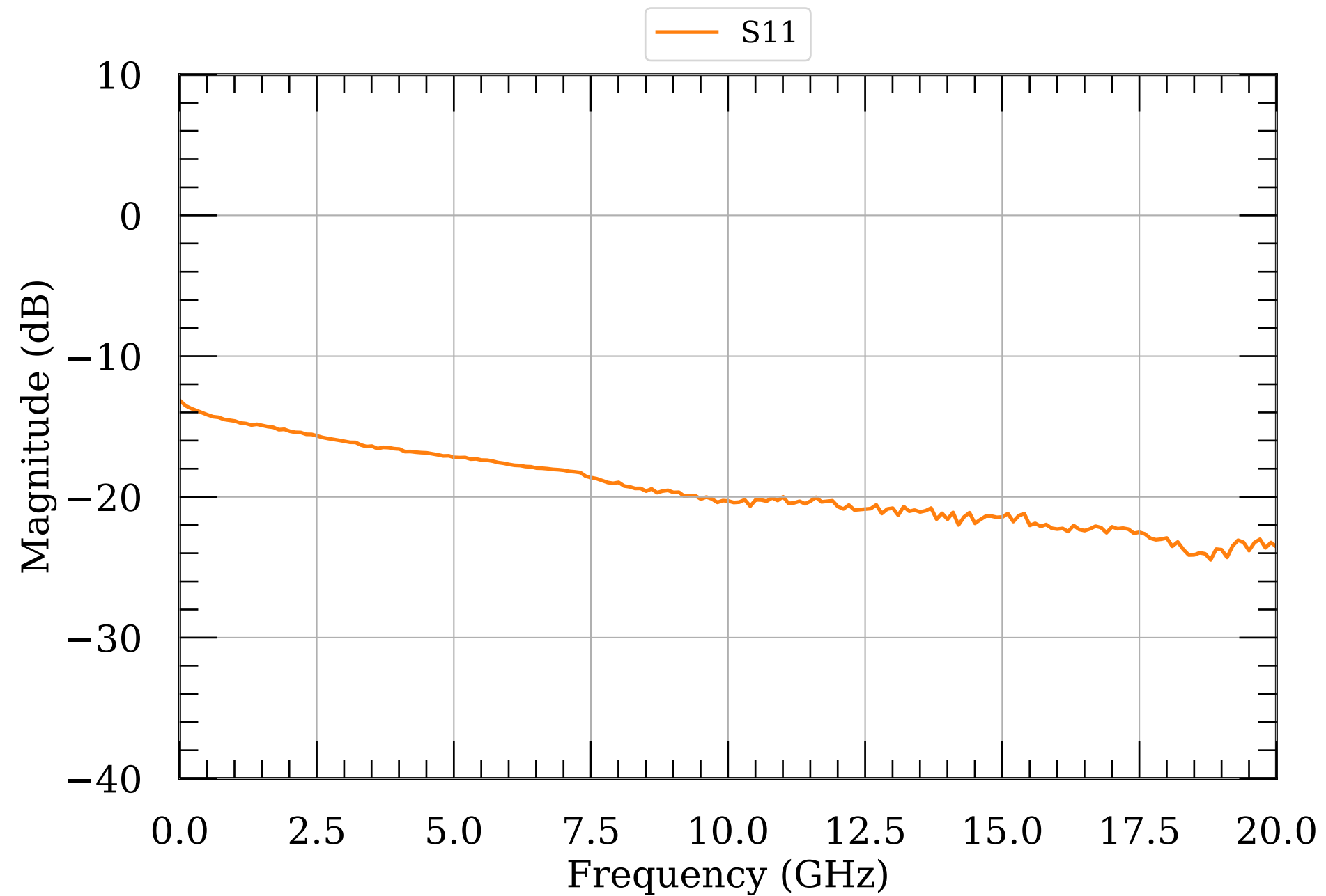
LNA S-params 265
