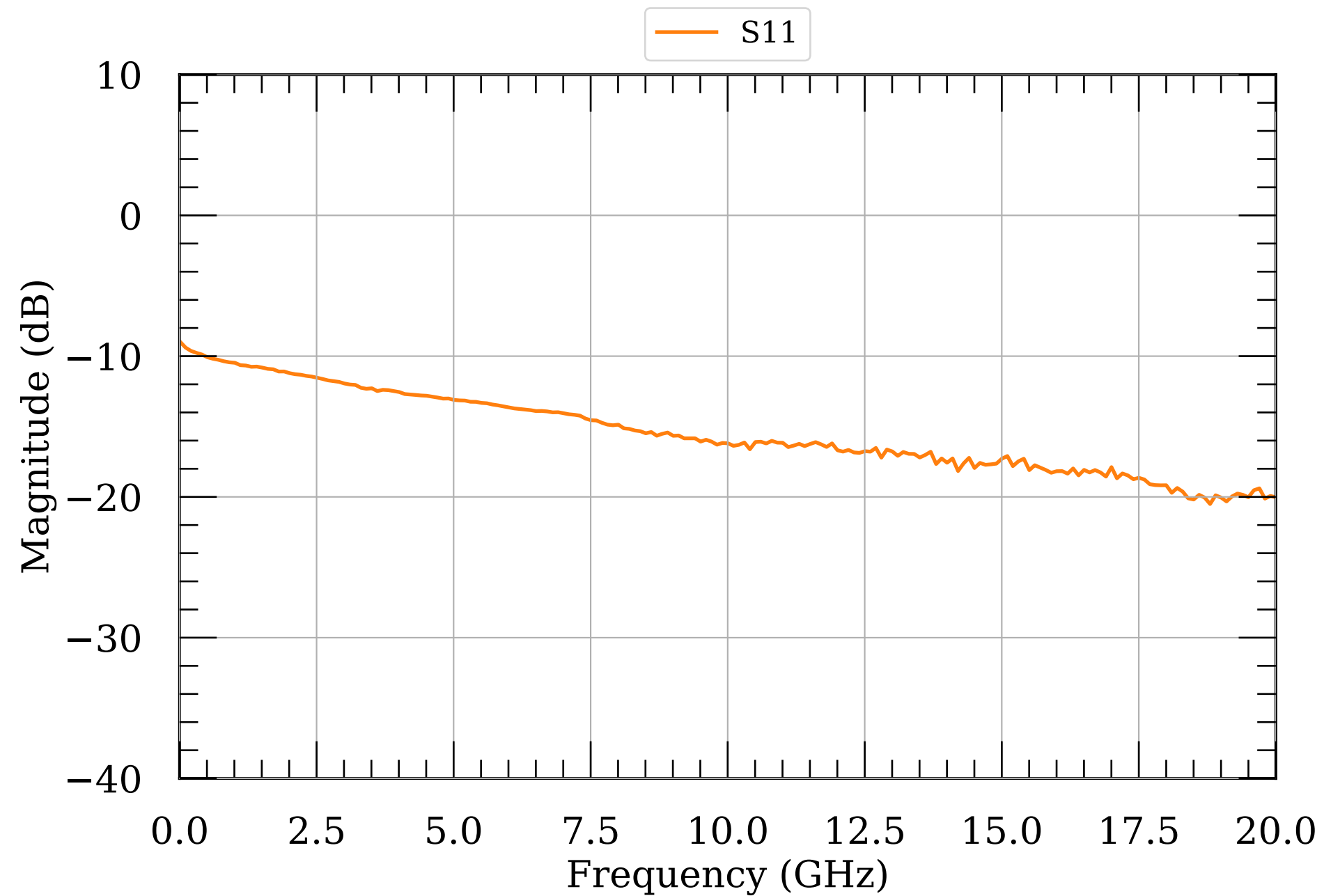
LNA S-params 280
