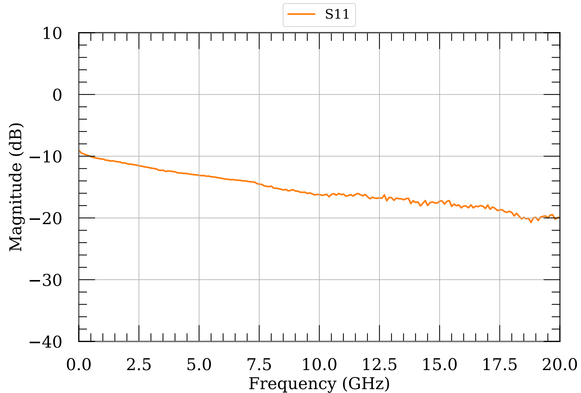
LNA S-params 285
