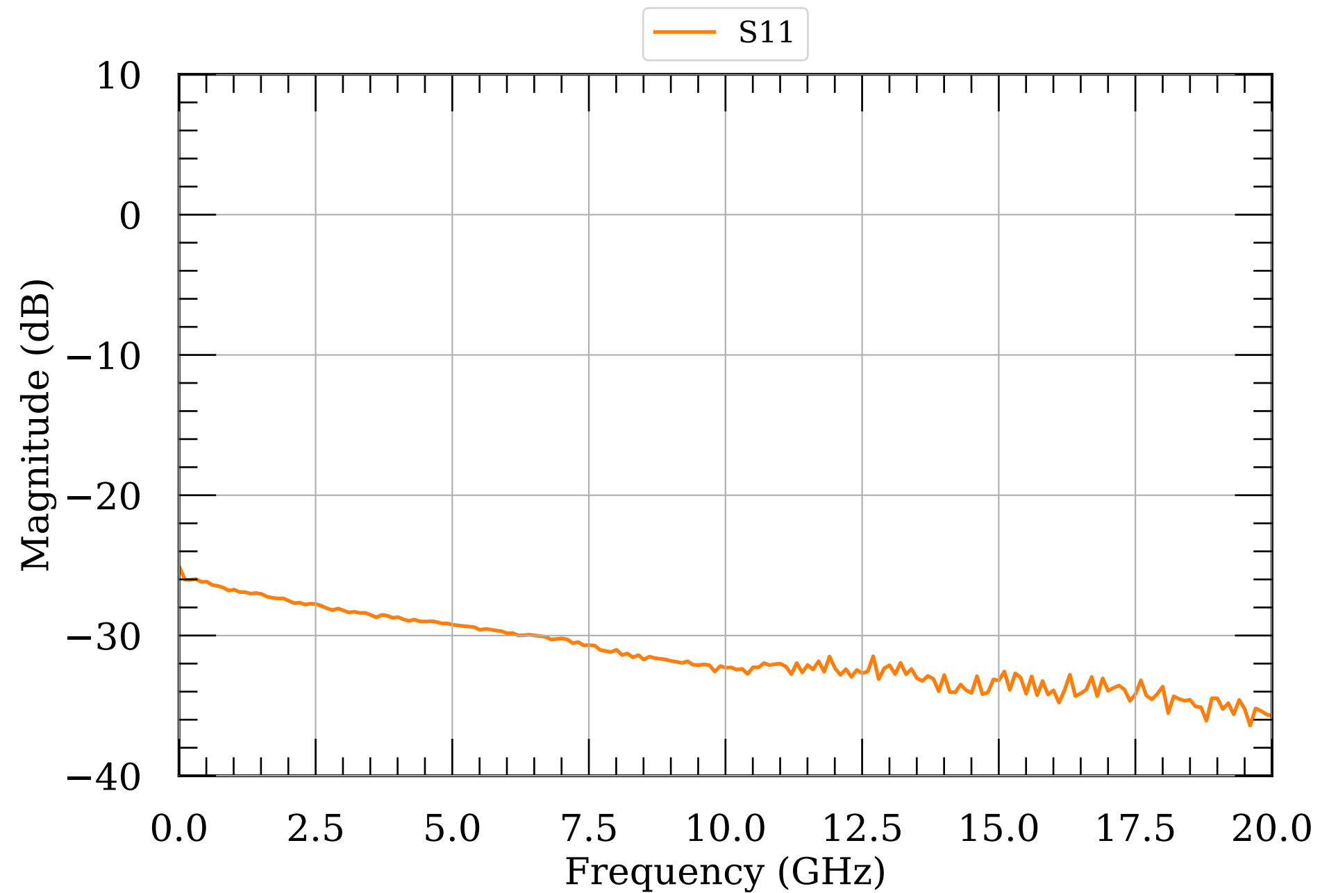
LNA S-params 290
