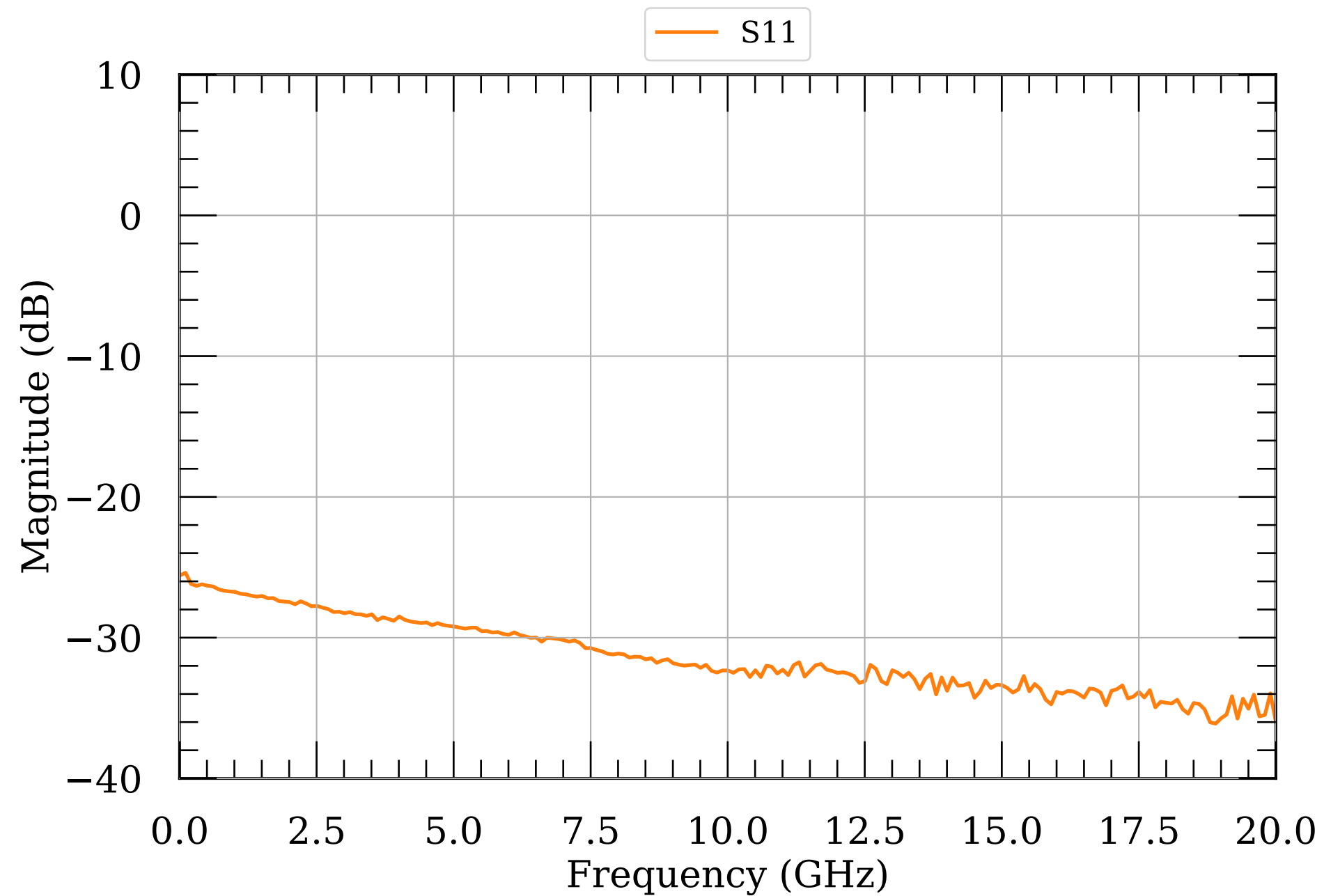
LNA S-params 295
