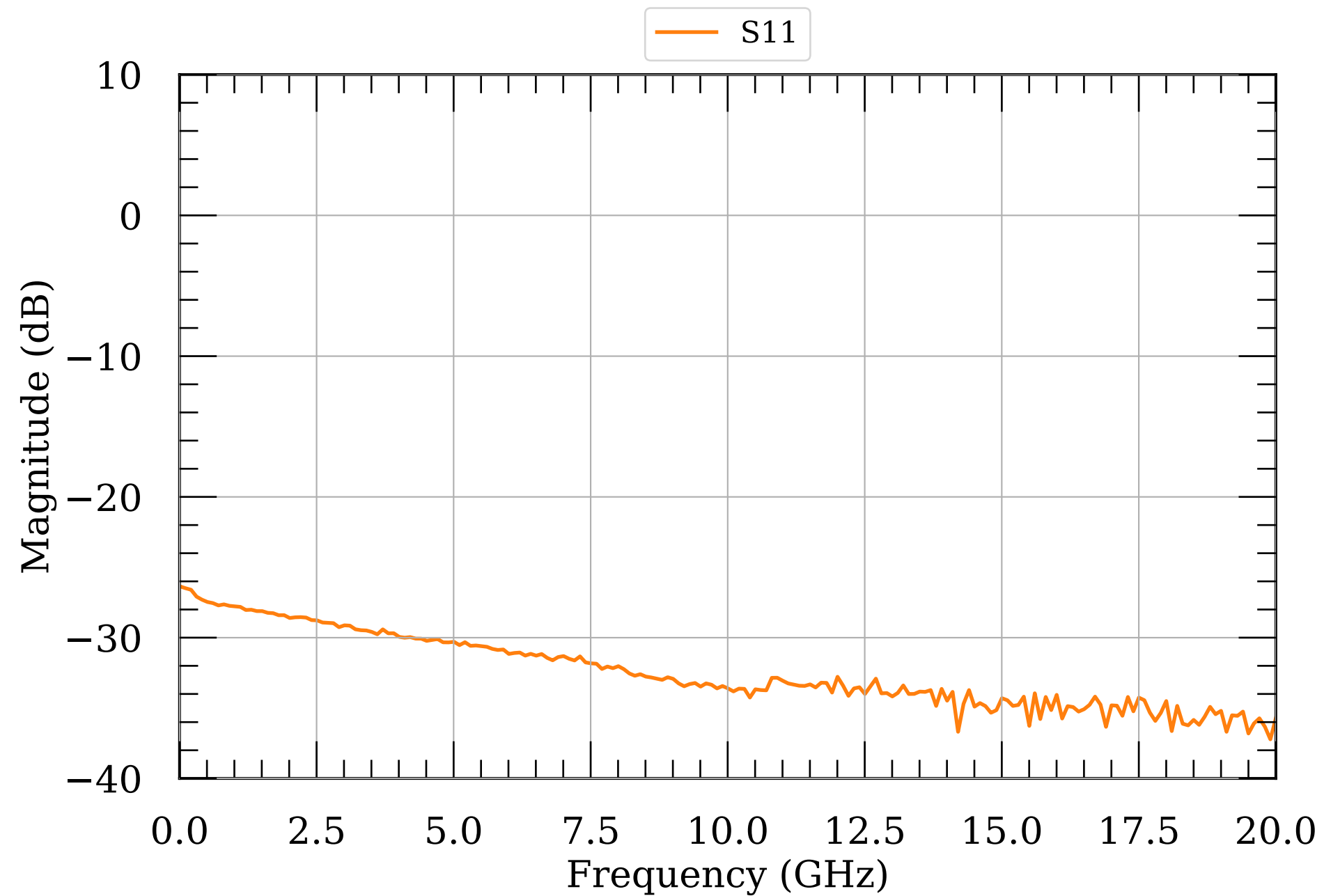
LNA S-params 30
