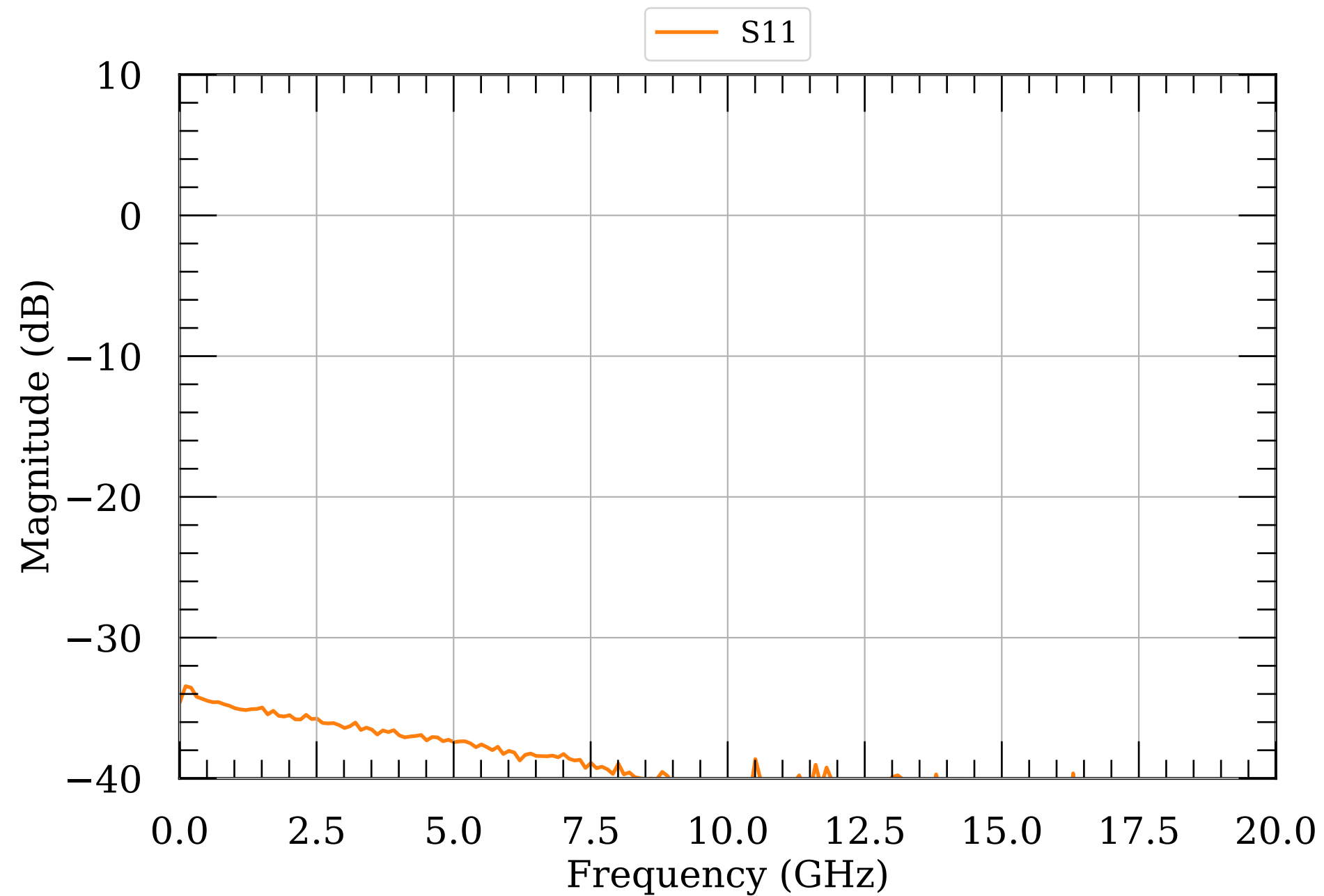
LNA S-params 310
