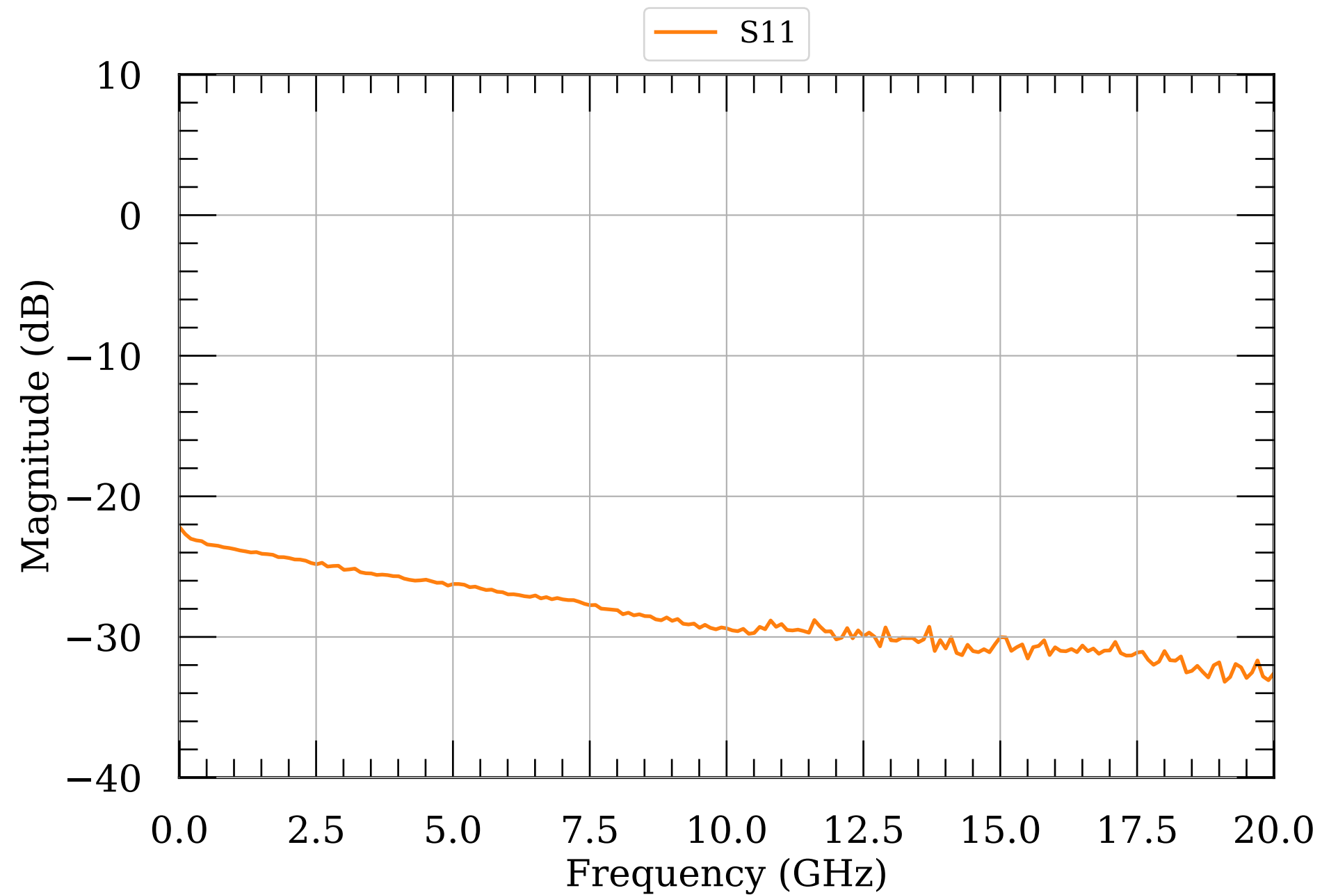
LNA S-params 55
