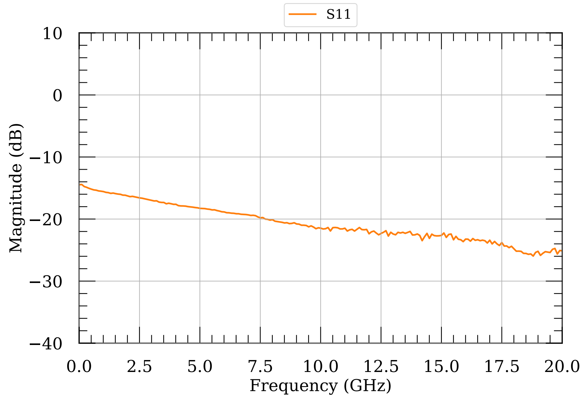
LNA S-params 60
