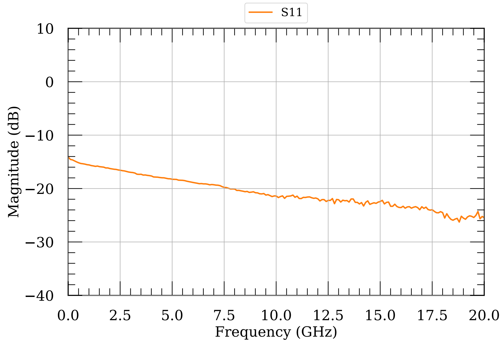
LNA S-params 65
