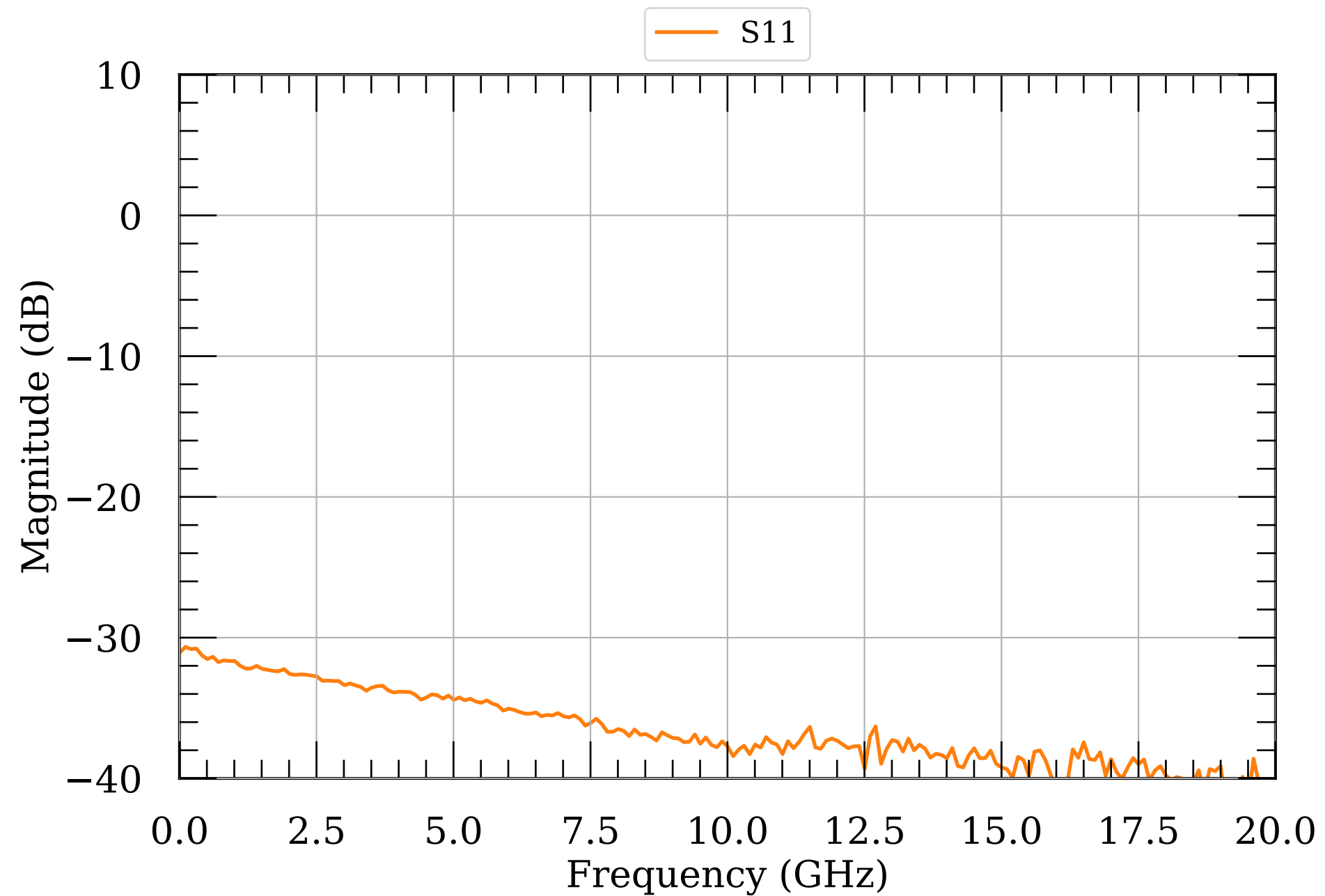
LNA S-params 70
