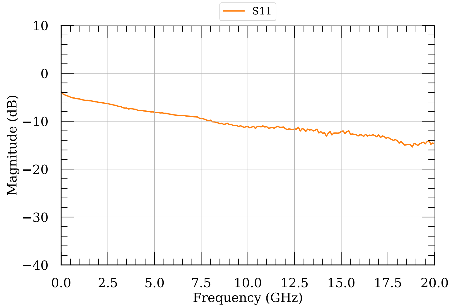
LNA S-params 80
