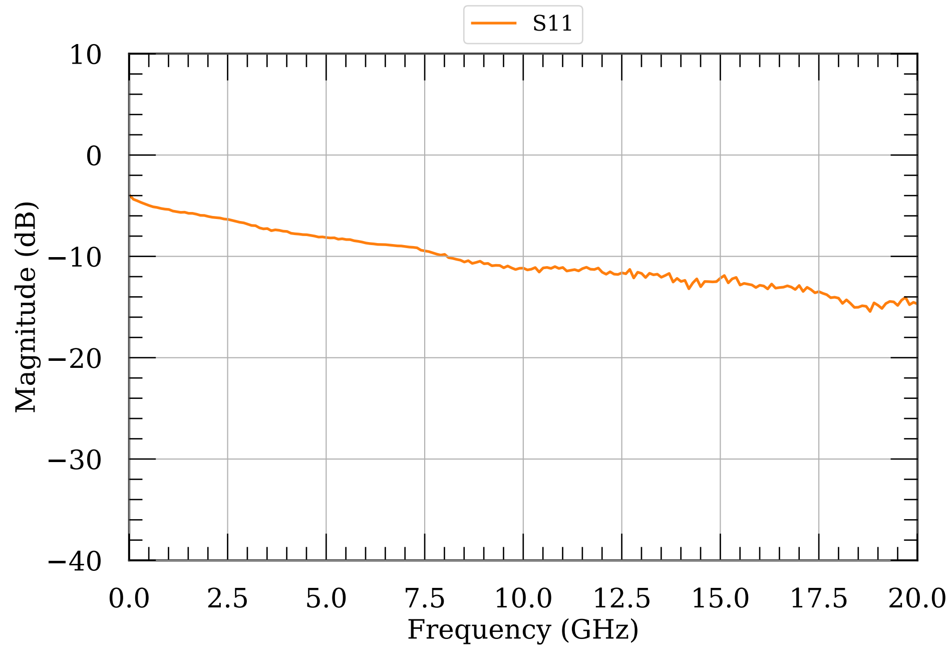
LNA S-params 85
