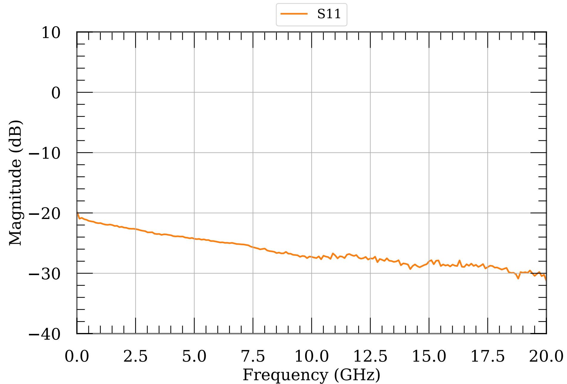
LNA S-params 95
