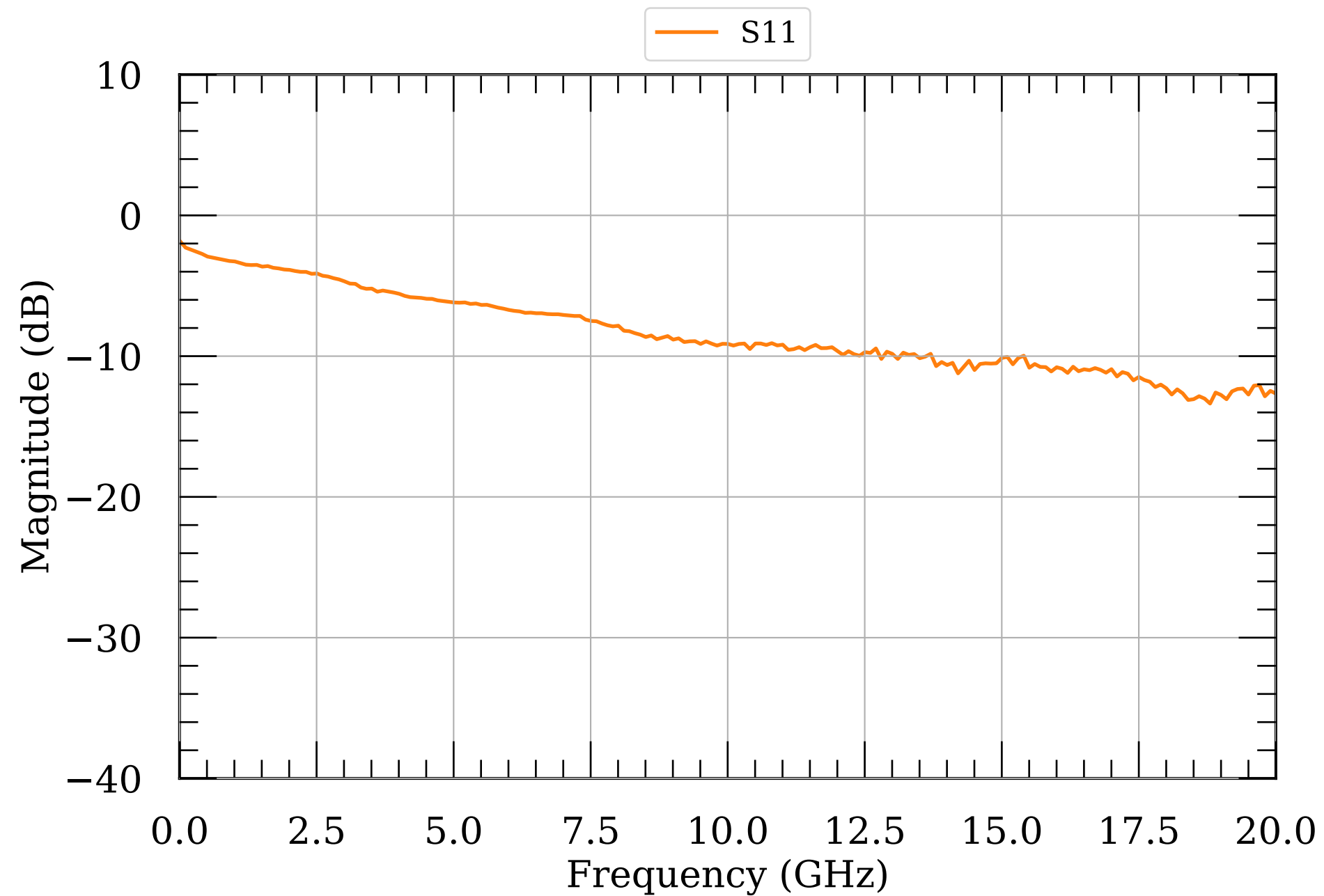
LNA S-params 0.5
