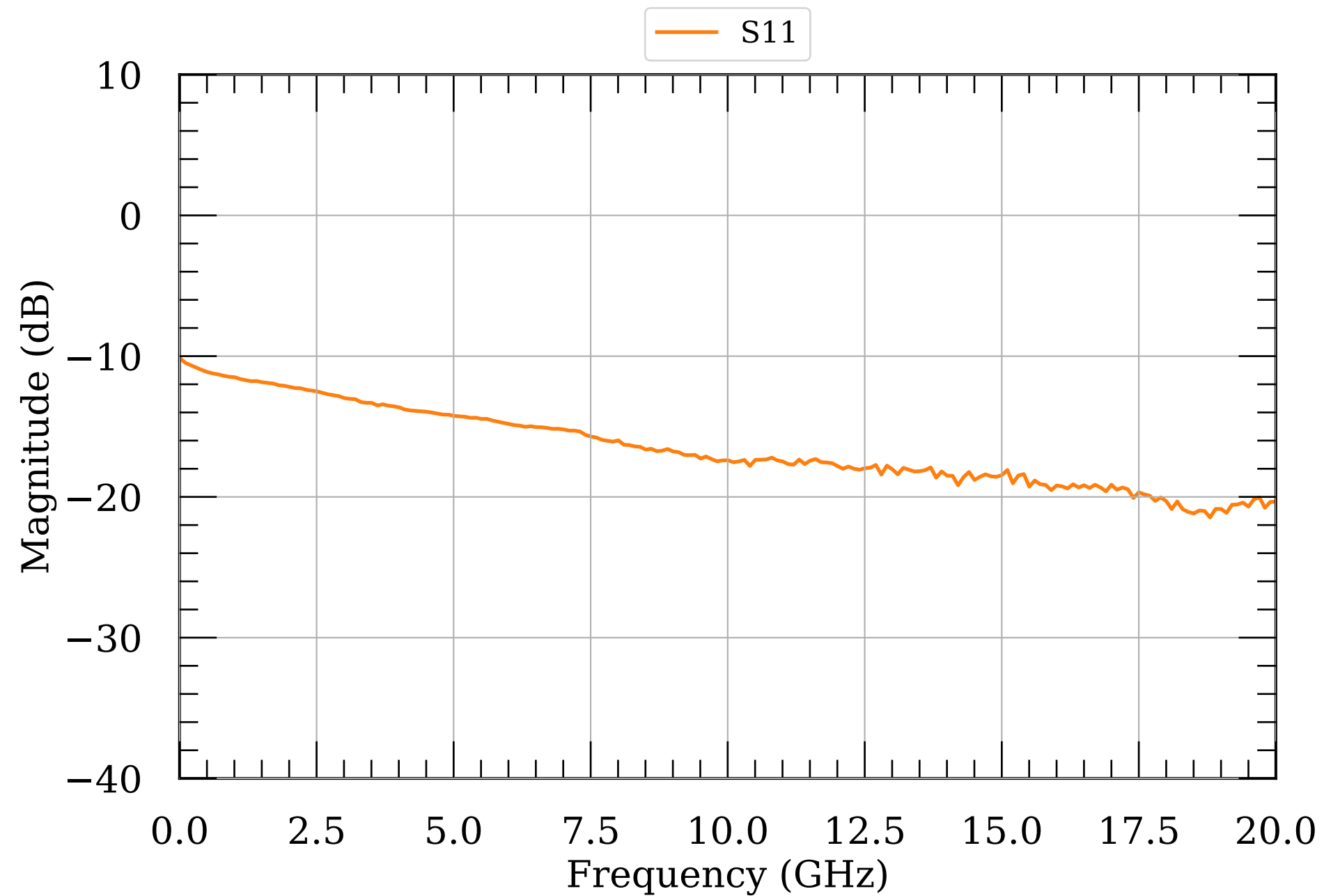
LNA S-params 2.0
