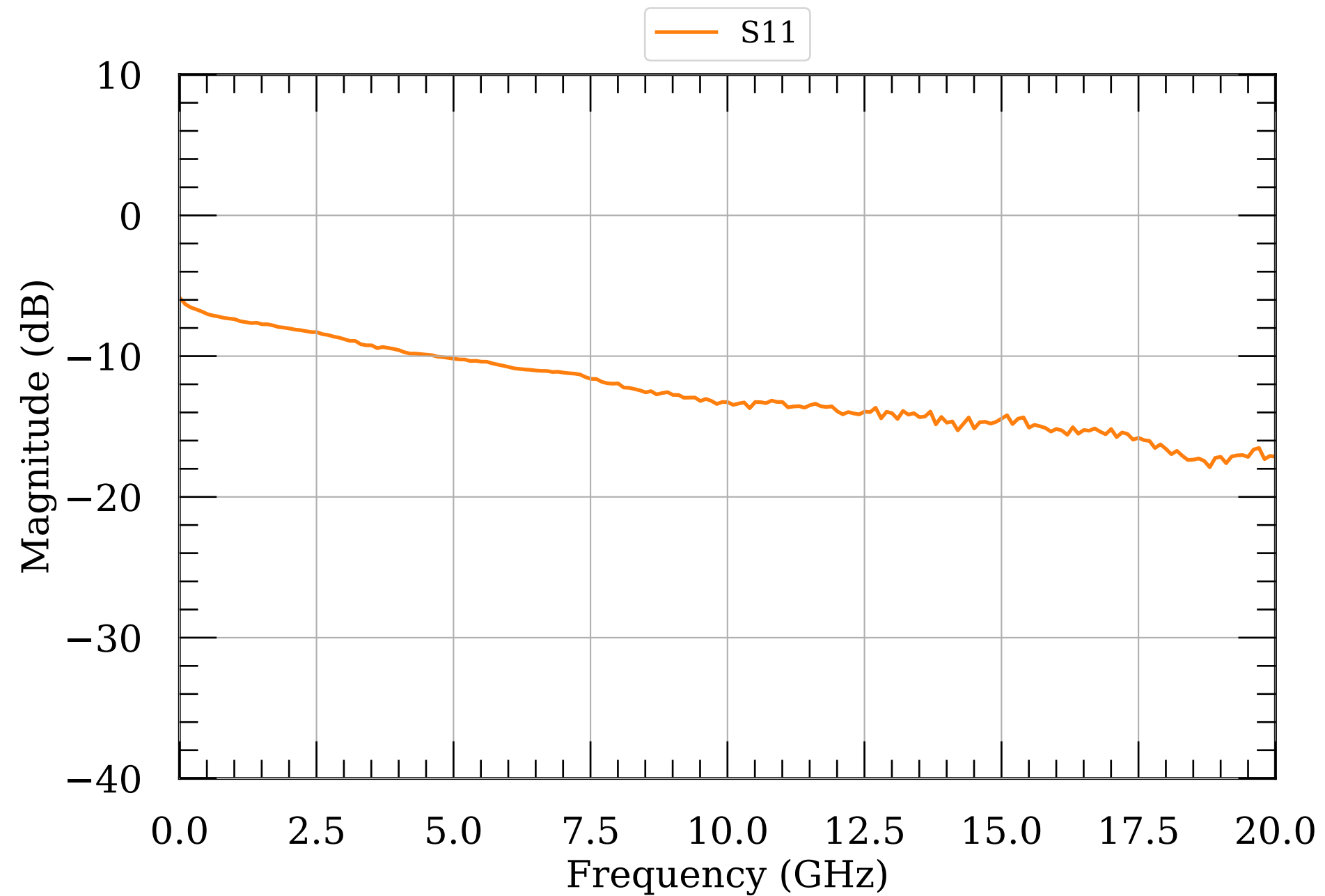
LNA S-params 4.5
