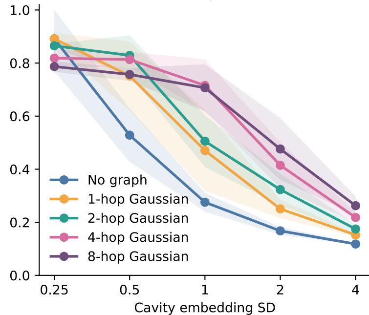
Cavity F1
