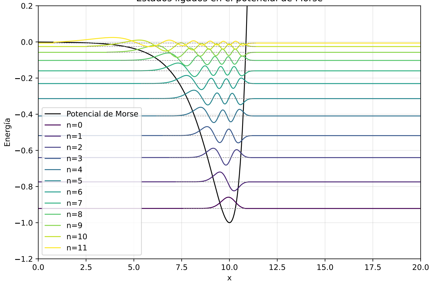
Estados ligados en el potencial de Morse
