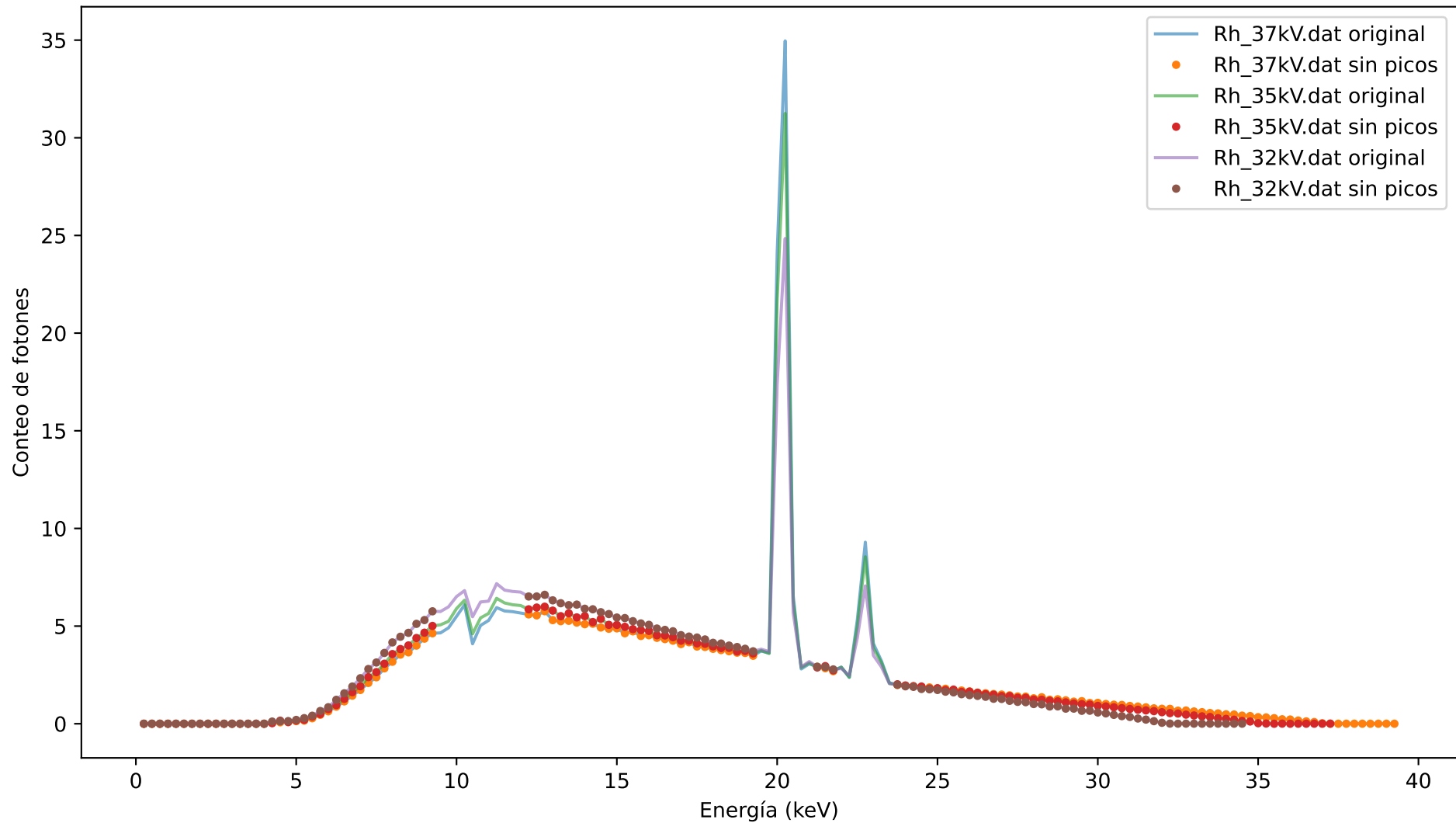
Ejemplos de espectros con picos removidos
