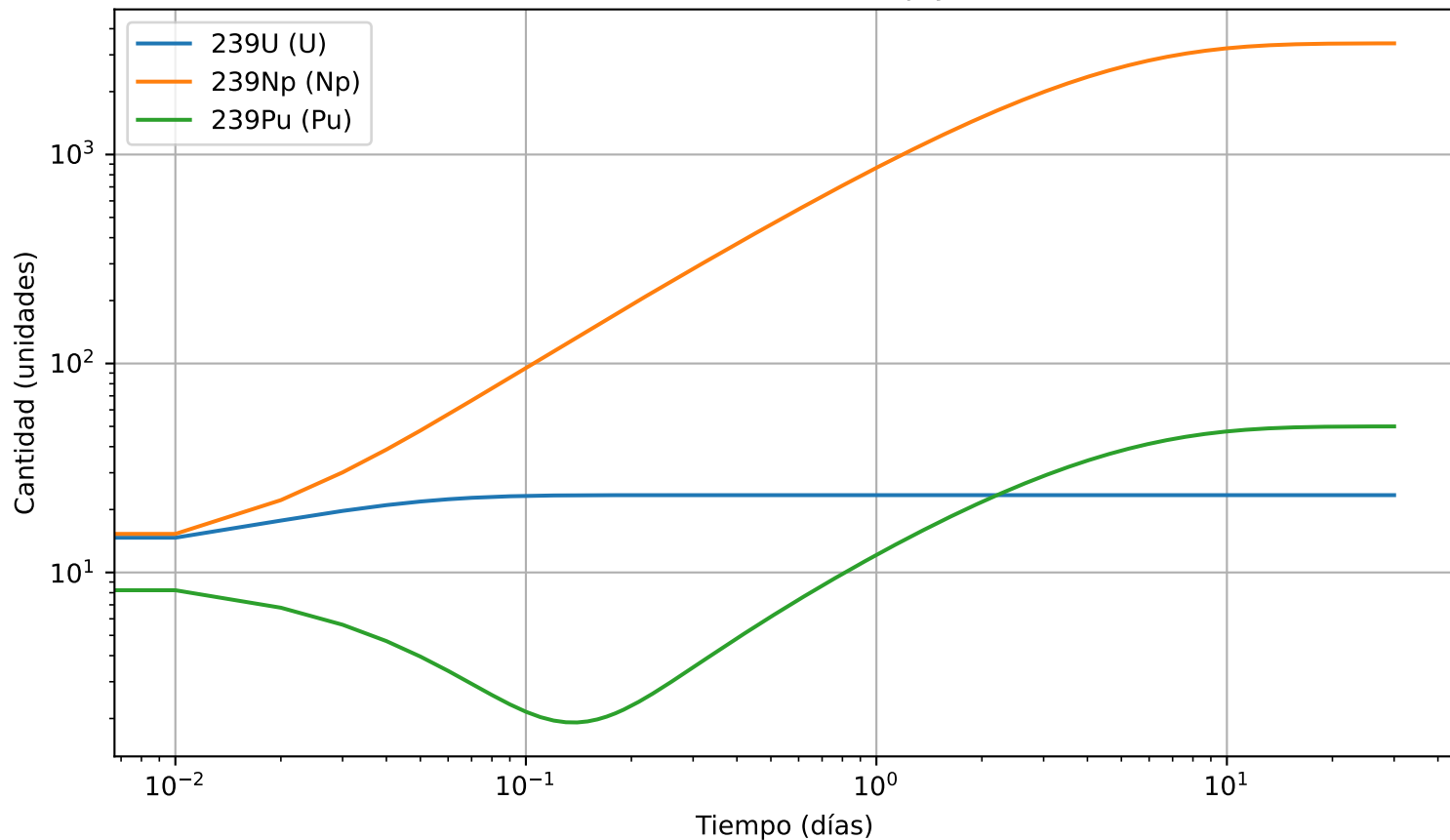
Evolución determinista de U, Np y Pu (30 días)
