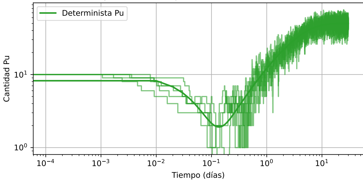
Trayectorias Gillespie SSA vs determinista (Pu)
