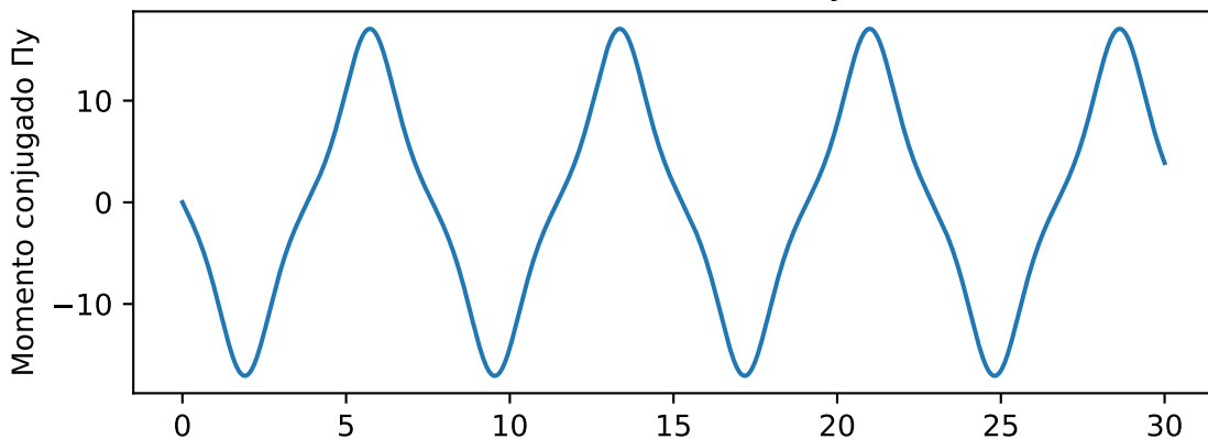
Conservación de \Pi_y
