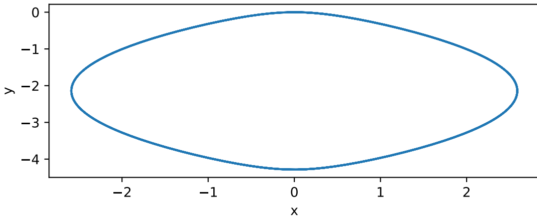
Trayectoria en el plano (x,y)
