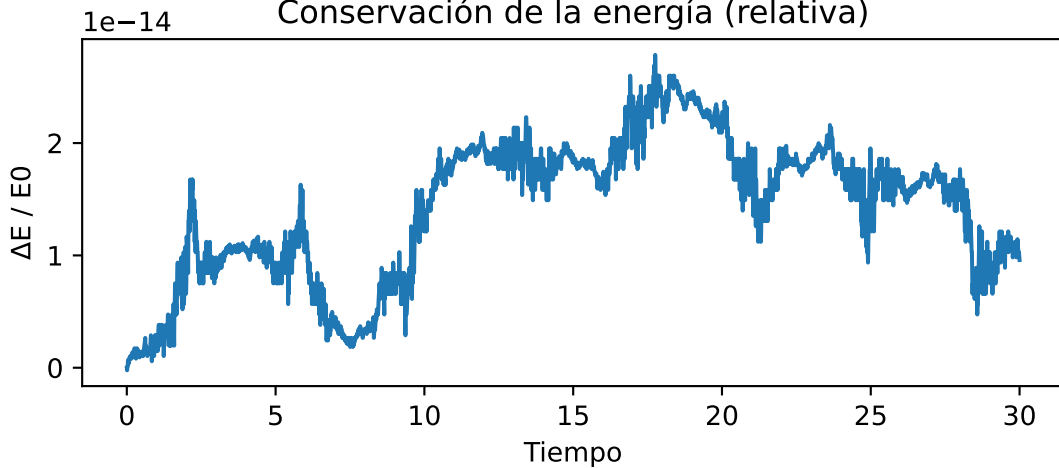
Conservación de la energía (relativa)
