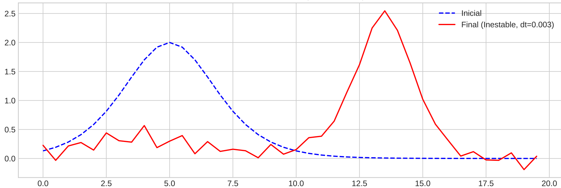
Simulación Inestable ( dt/dx^3 = 0.02 )
