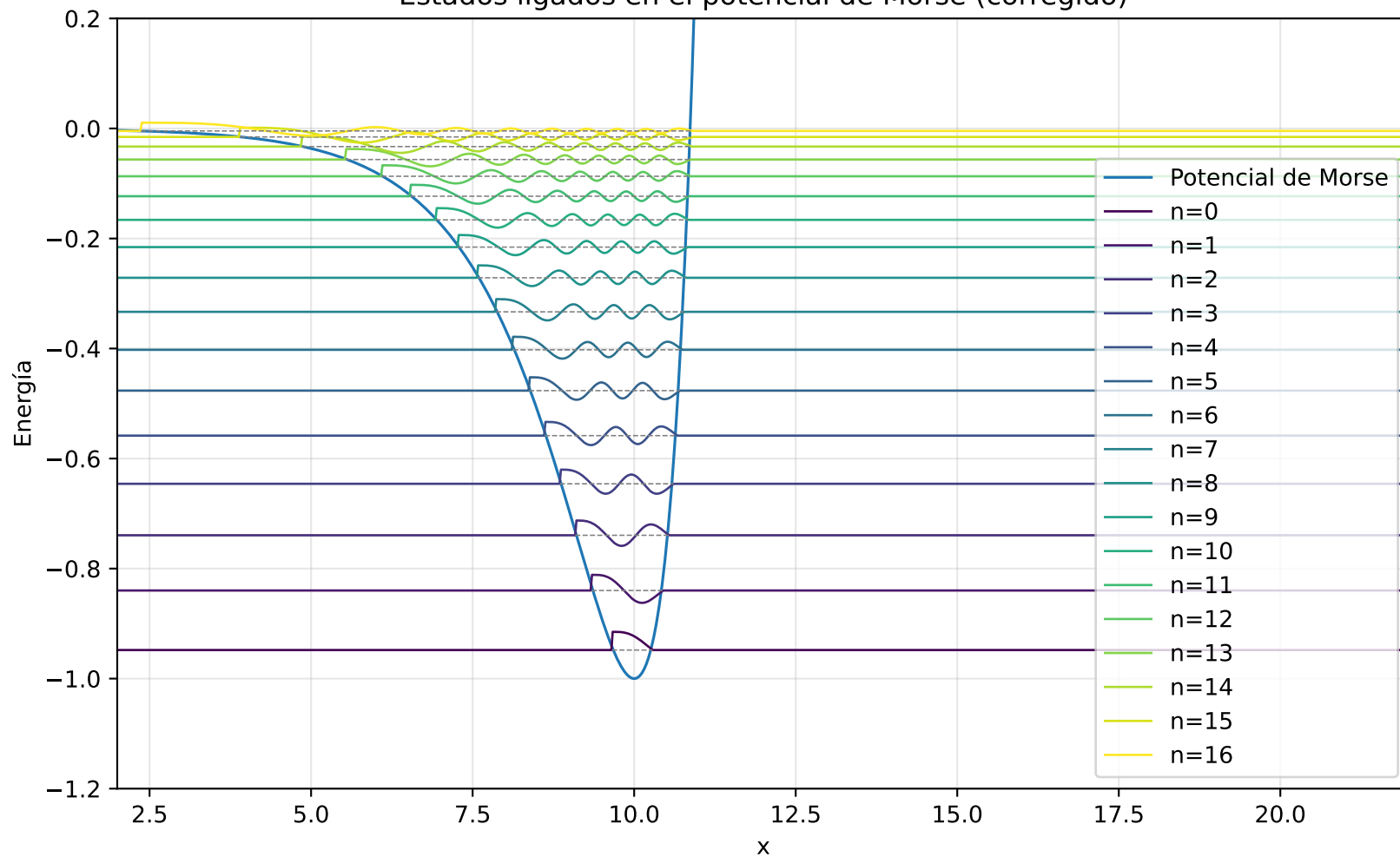
Estados ligados en el potencial de Morse (corregido)
