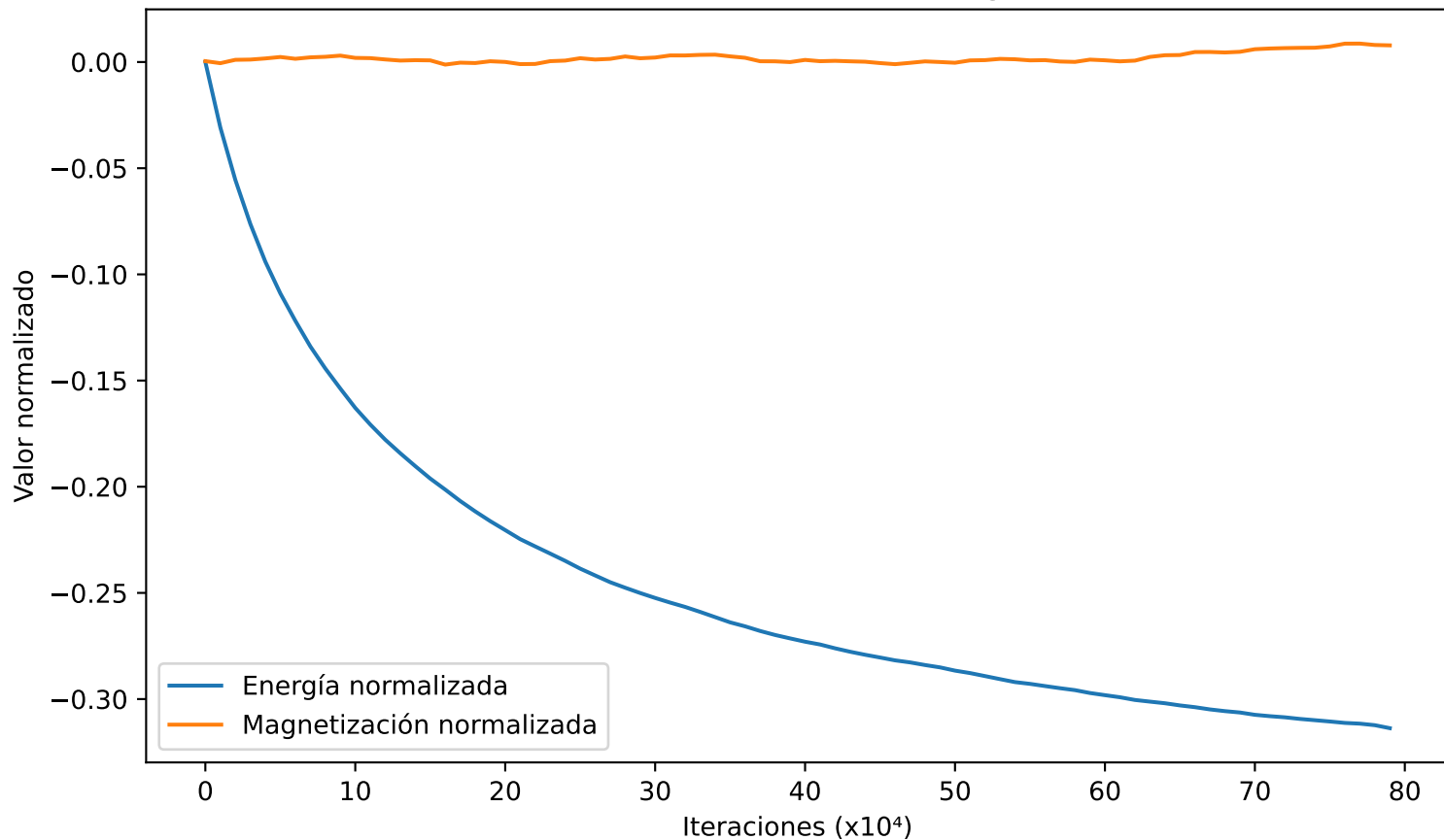
Evolución del modelo de Ising 2D
